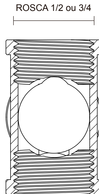
CORTE A-A
