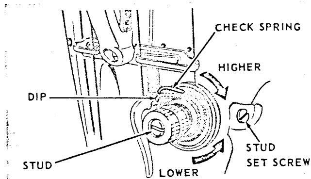
Fig. 55. Check Spring
