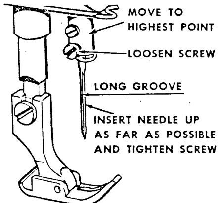
Fig. 12. Machine 281-23
