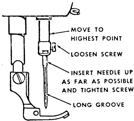
Fig. 9. Machine 281-5
