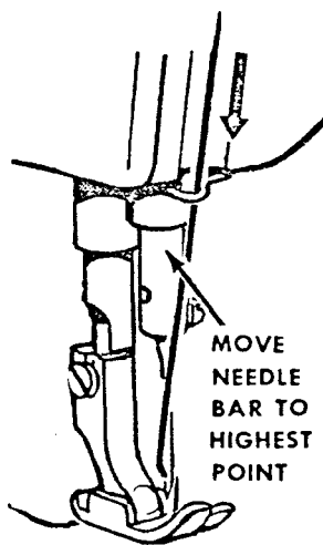
Fig. 16. Machines 281-6 and 281-20 281-30
