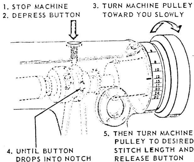
Fig. 29. Machine 281-5
