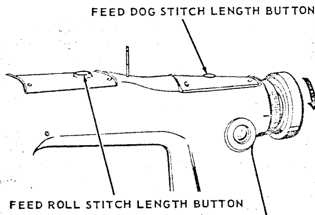
281-30 Fig. 31. Machines 281-20 and 281-23
