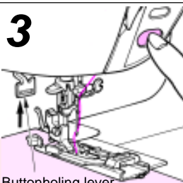
Buttonholing lever Lever de boutonnière Palanca del soporte del prensatelas de ojales.
