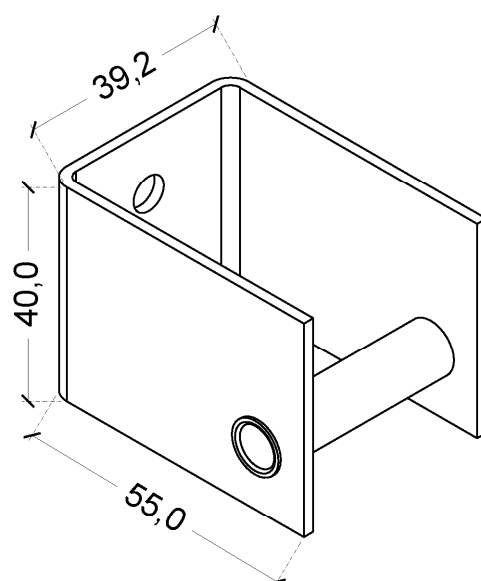
Halter mit Einhängbolzen Typ 2
