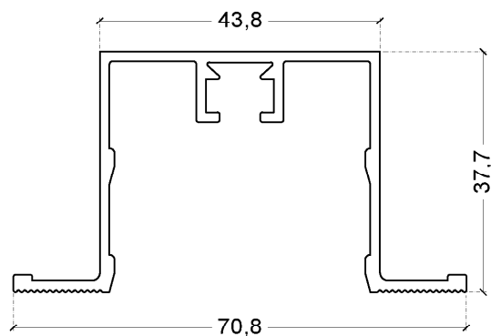
Profil E97103 oder Profil 33413
