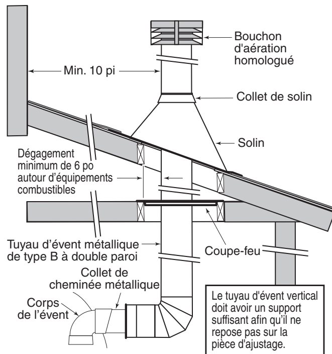
Figure 18. – L'installation de tuyau de conduit en métal typique - É.-U. (Verticale- la Pression Négative)
