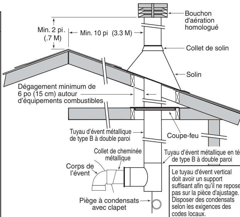
Figure 19. – L'installation de tuyau de conduit en métal typique - Canada. (Verticale - la Pression Négative)
