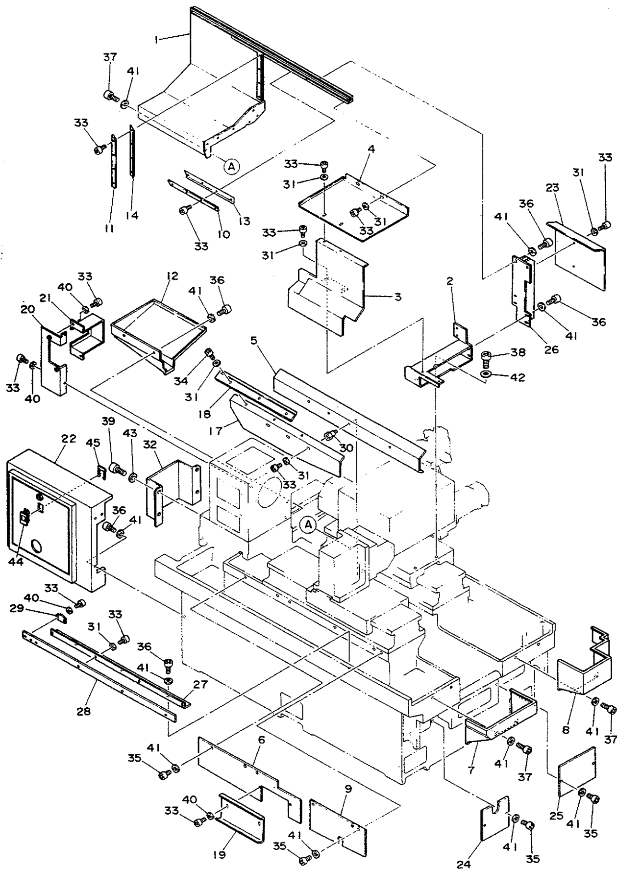
オイルガード-3/3 Fig.59 OIL GUARD-3/3
