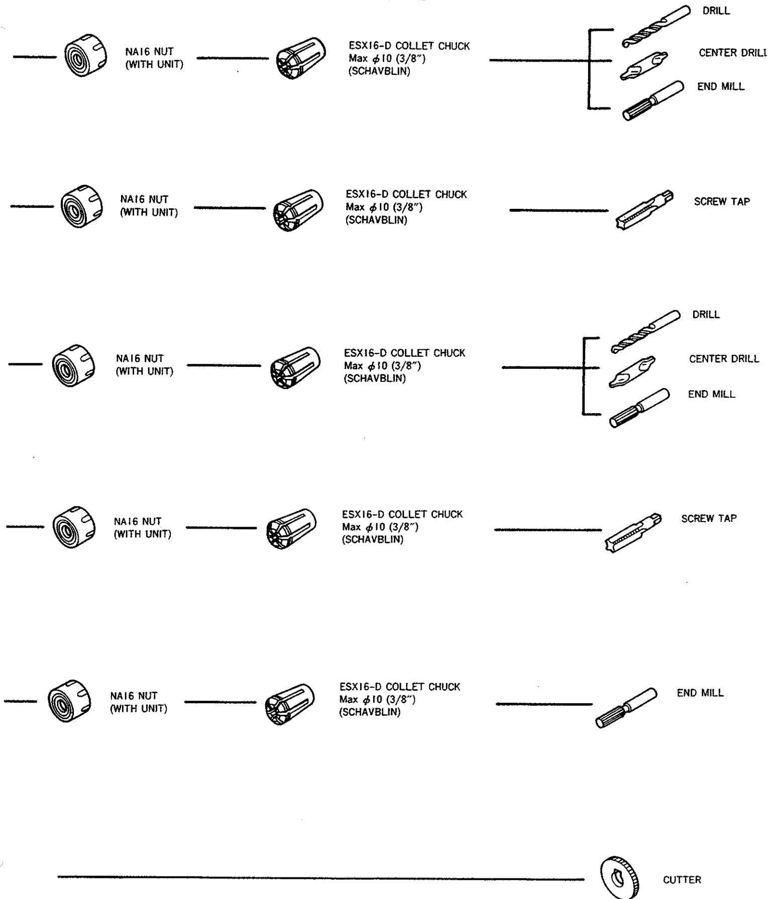
リボルビングツールシステム図 (輸出) Fig.16 REVOLVING TOOL SYSTEM (FOR EXPORT)
