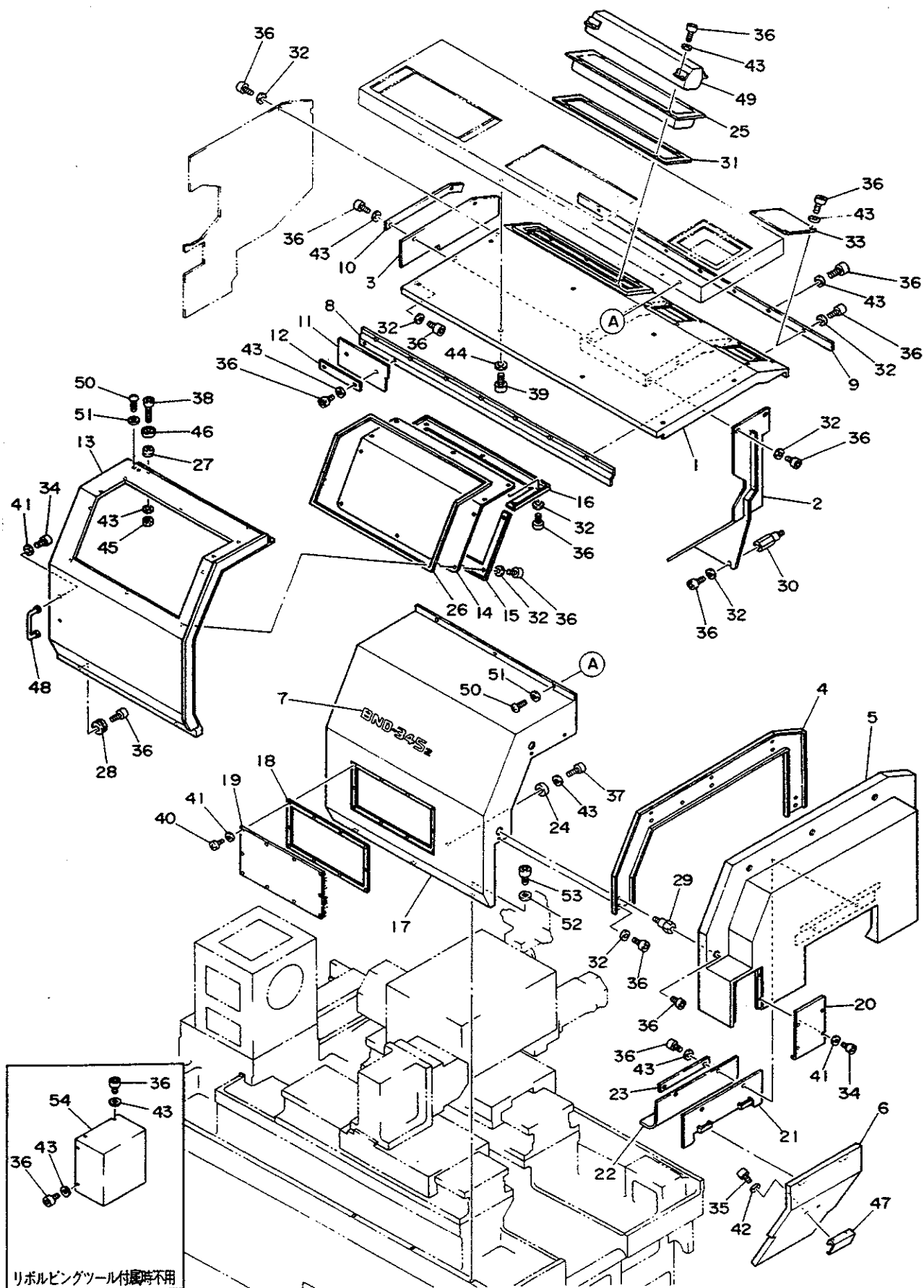
オイルガード-2/3 Fig.58 OIL GUARD-2/3
