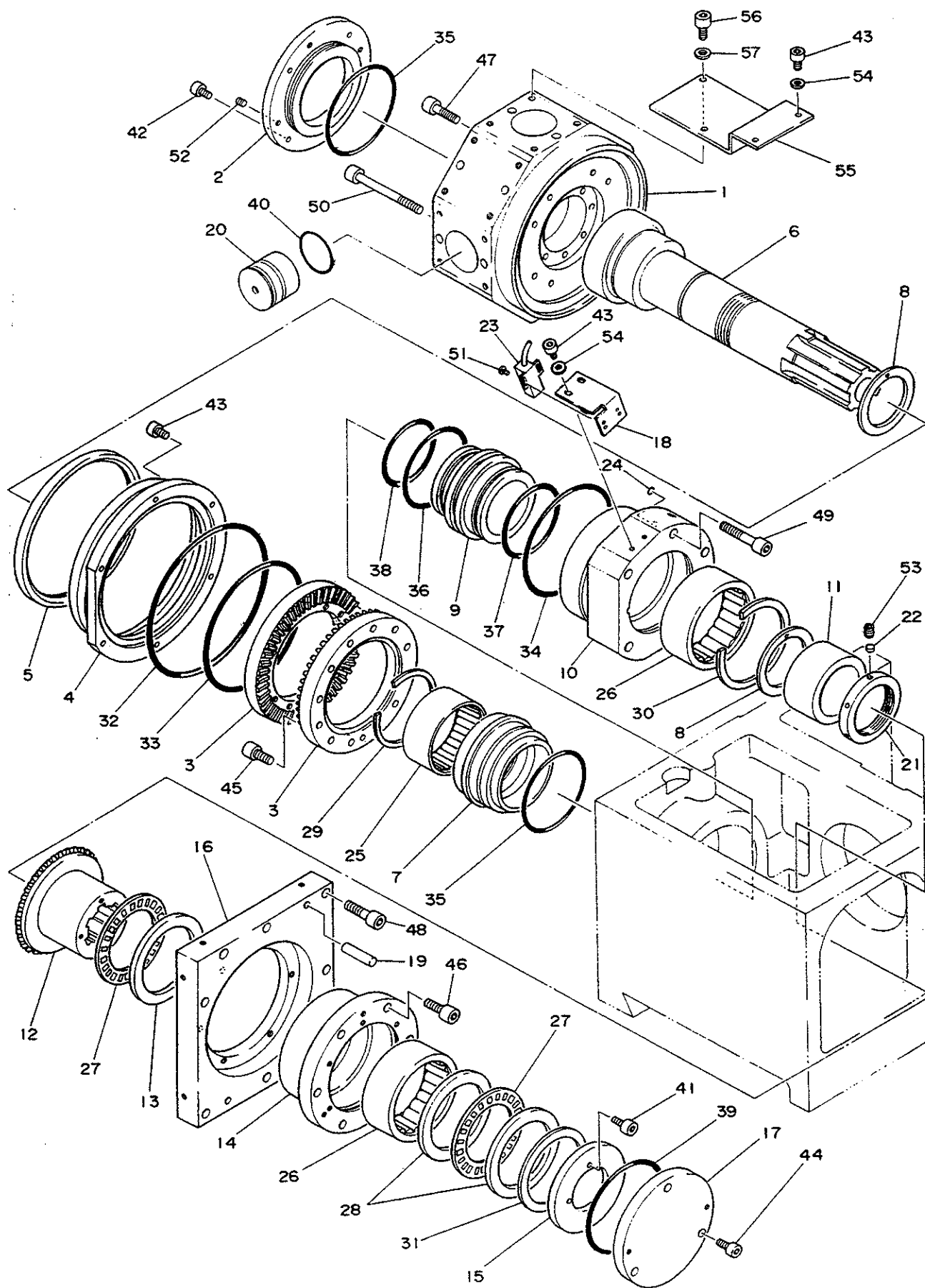
メインタレットスライド-3/7 Fig.49 MAIN TURRET SLIDE-3/7
