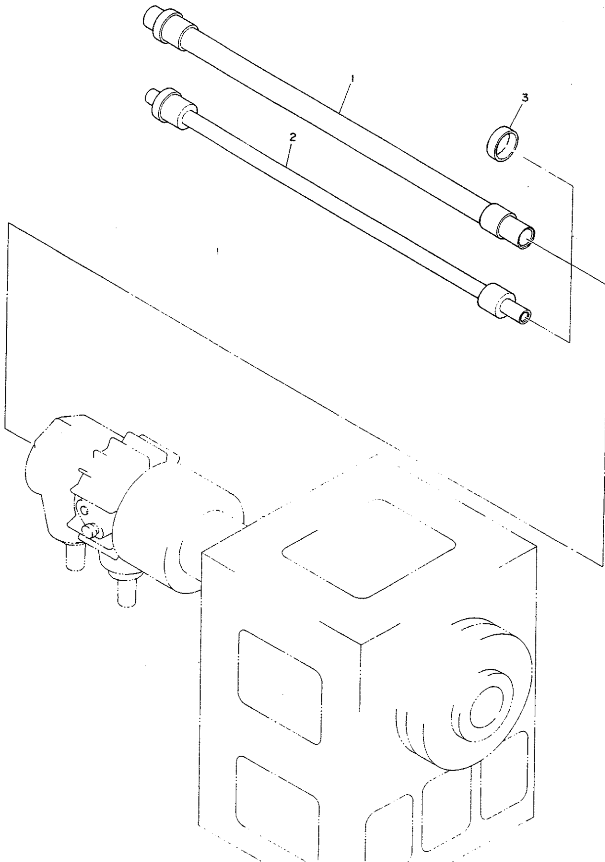
Fig.103 フィラチューブアッセンブリ (ASR.F-34M) FILLER TUBE ASSEMBLY (ASR.F-34M)
