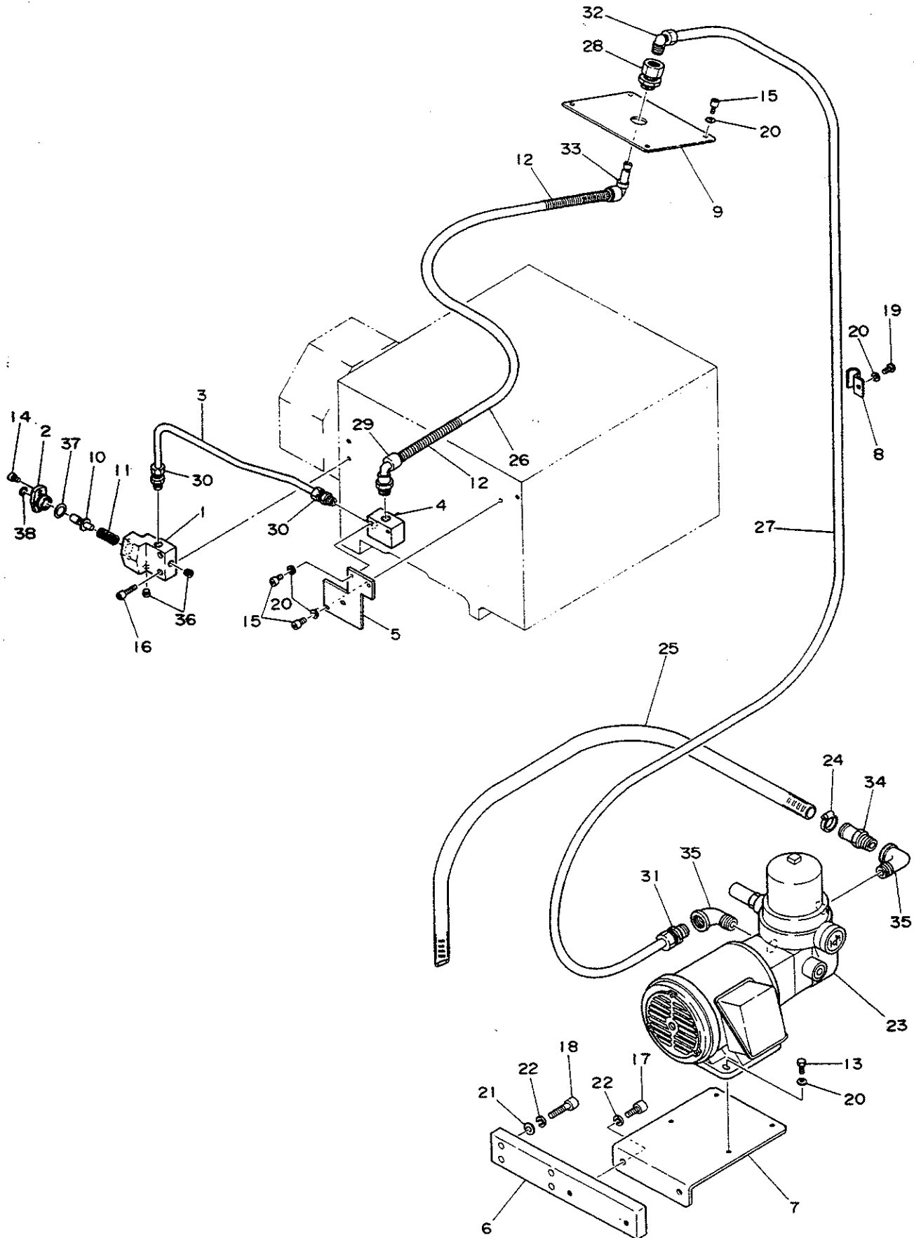
メインハイプレッシャークーラント Fig.62 MAIN HIGH PRESSURE COOLANT
