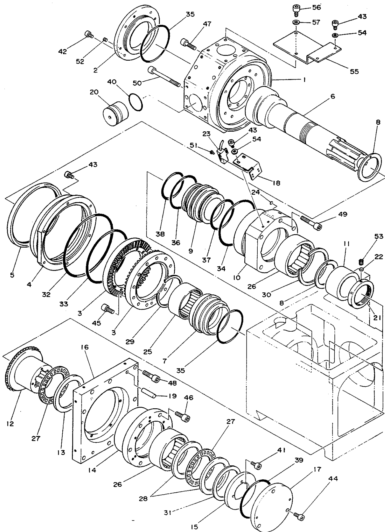
メインタレットスライド-3/7 Fig.49 MAIN TURRET SLIDE-3/7
