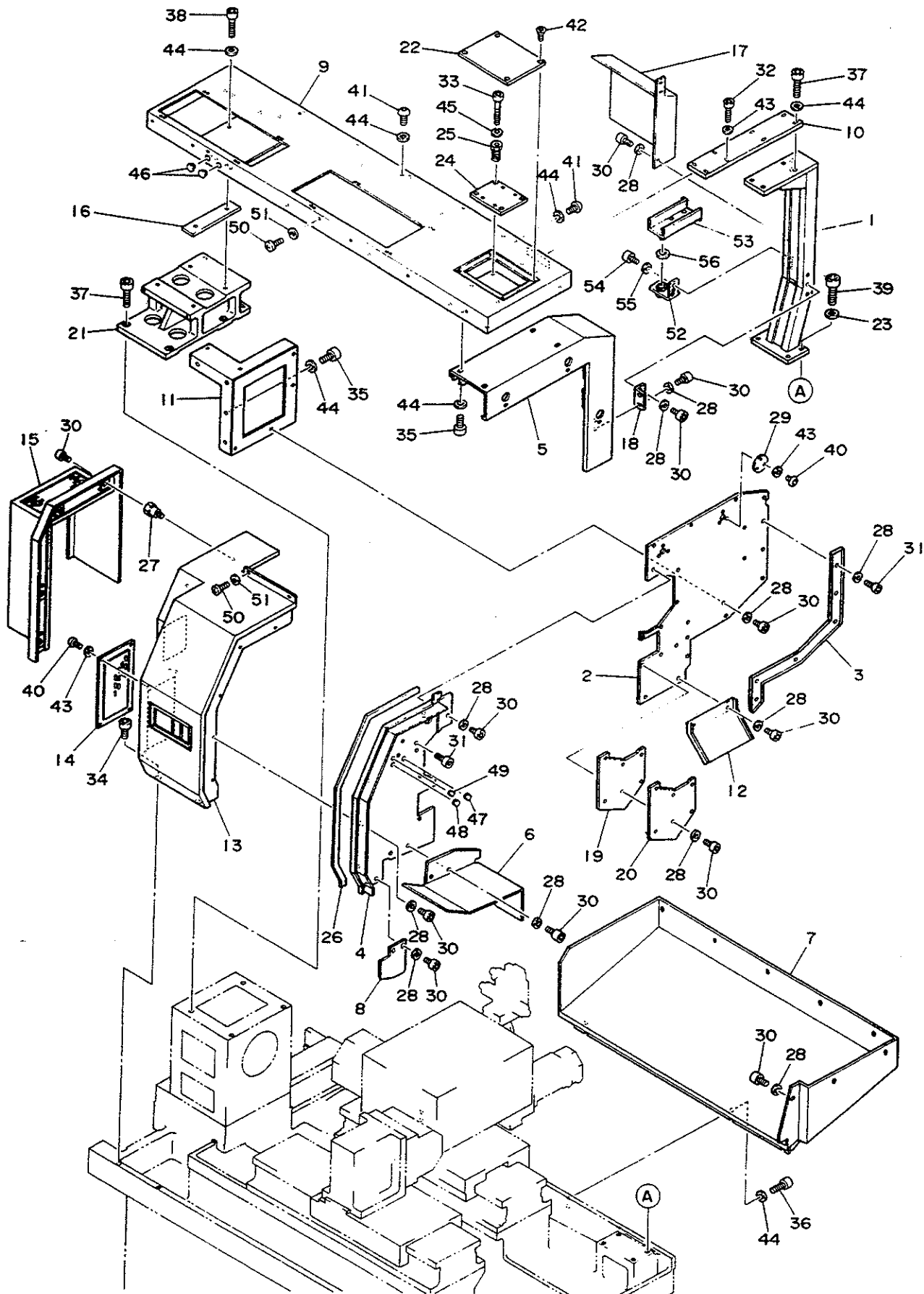
オイルガード-I/3 Fig.57 OIL GUARD-I/3
