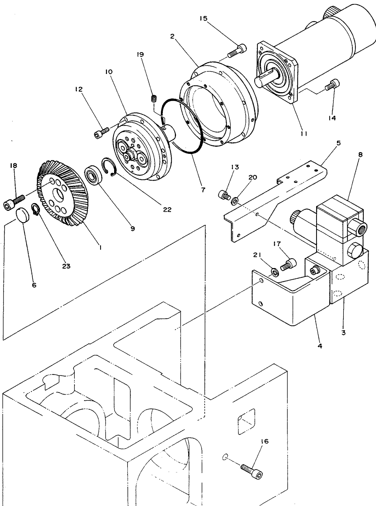
メインタレットスライダー4/7 Fig.50 MAEN TURRET SLIDE-4/7
