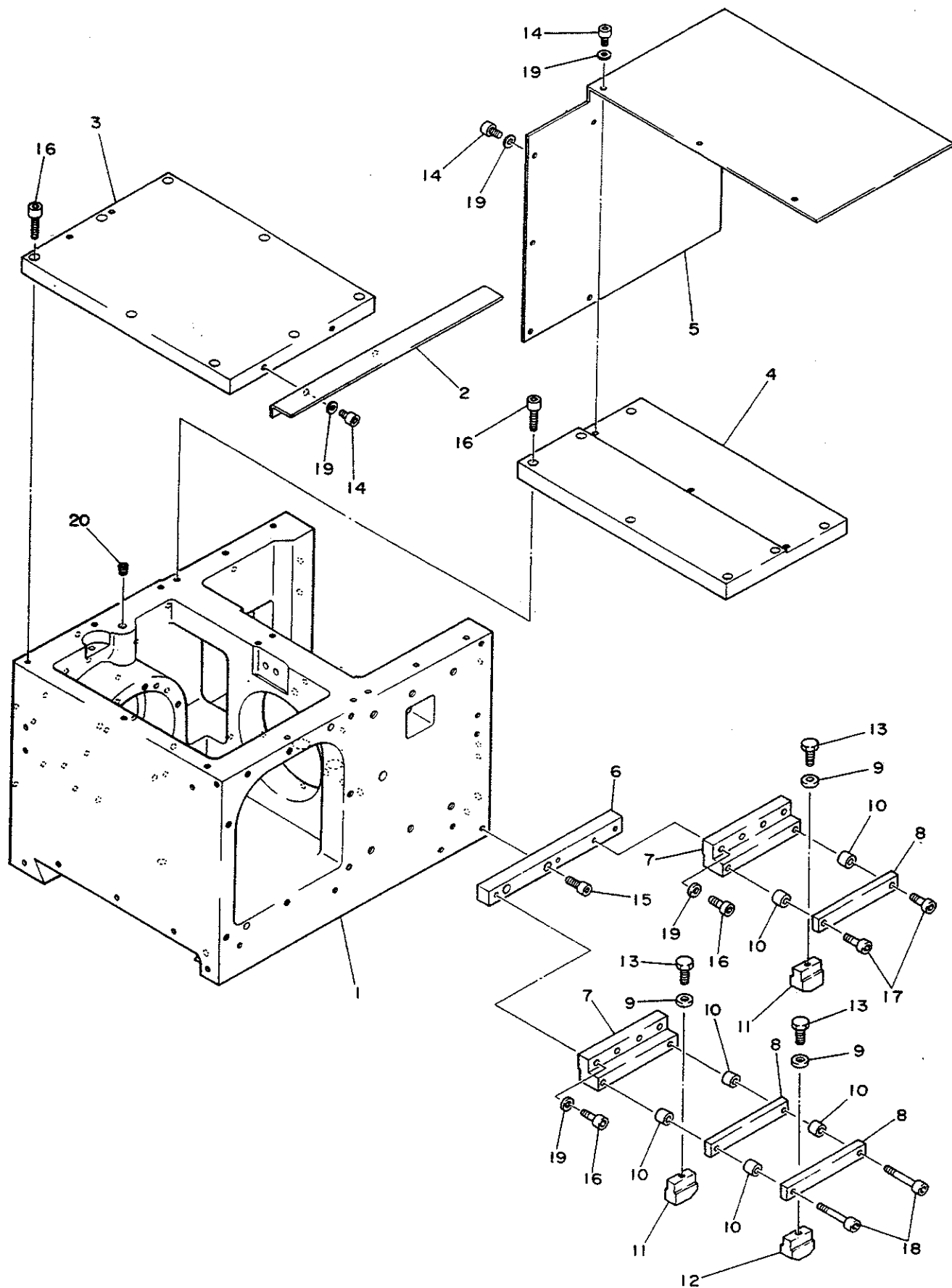
メインタレットスライド-1/7 Fig.47 MAIN TURRET SLIDE-1/7
