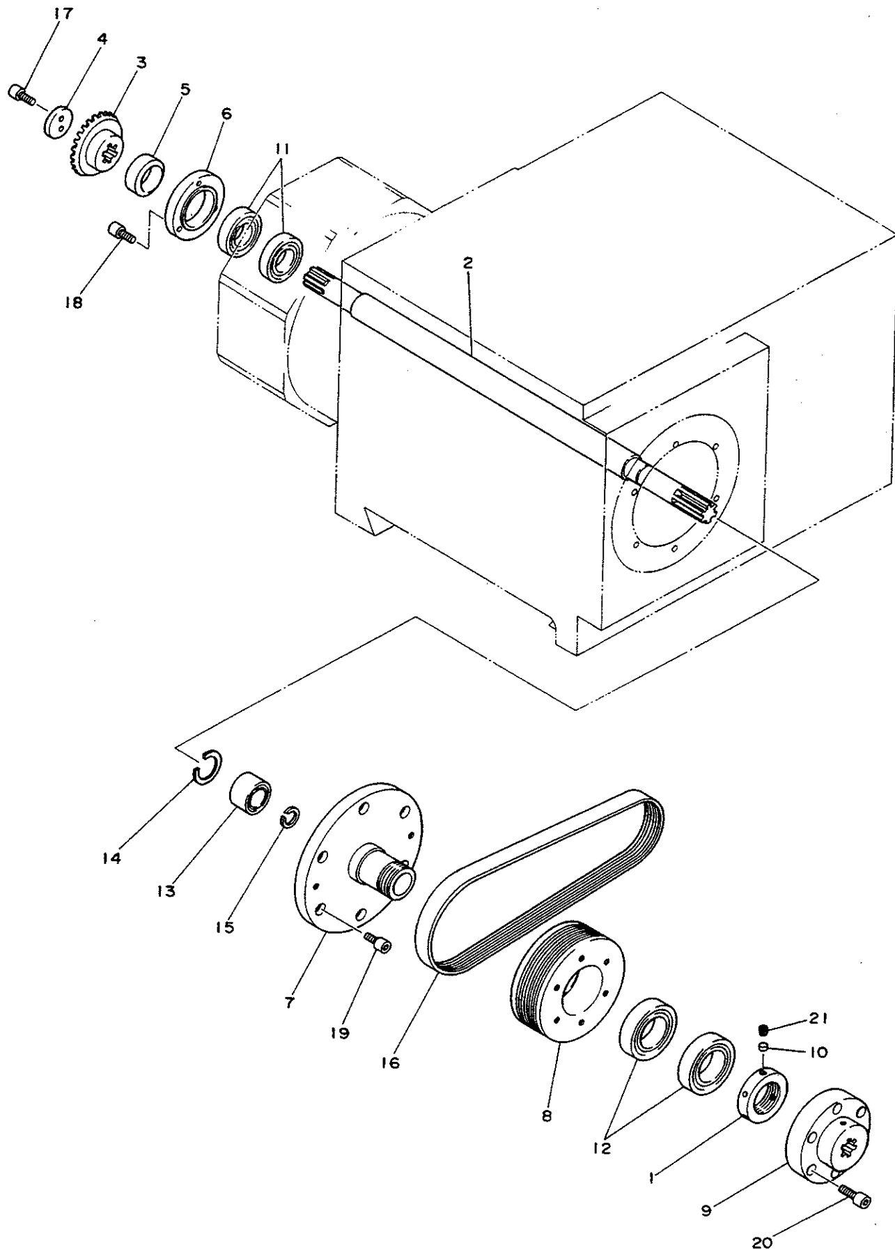
リボルビングツールドライビングユニット-2/2 Fig.93 REVOLVING TOOL DRIVING UNIT-2/2
