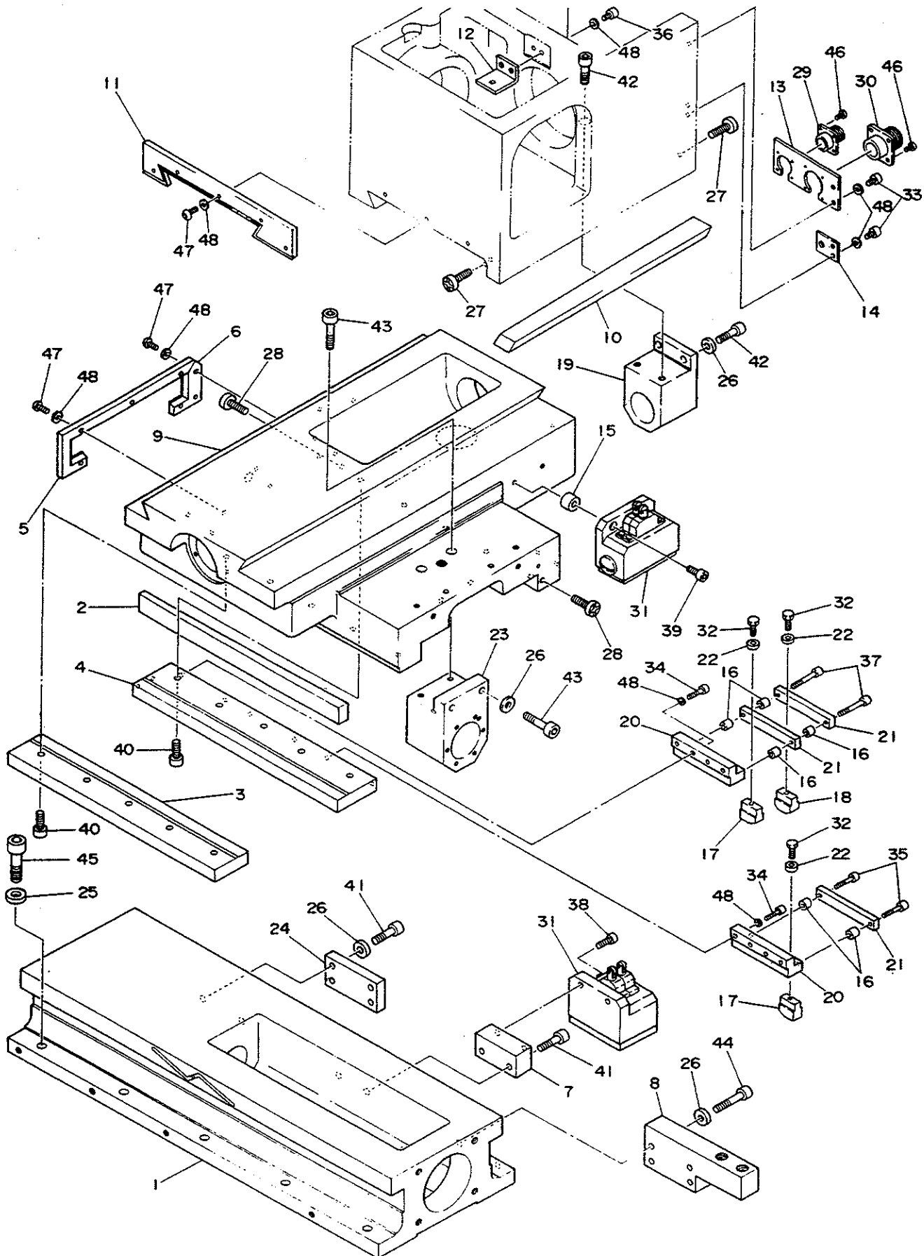
メインタレットスライド-2/7 Fig.48 MAIN TURRET SLIDE-2/7
