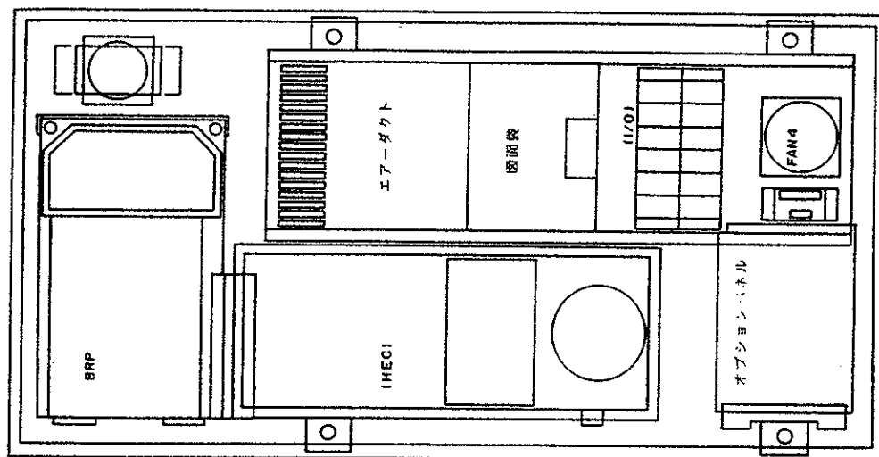
NCボックス内機器配置図 Fig.97 LAYOUT OF NC BOX
