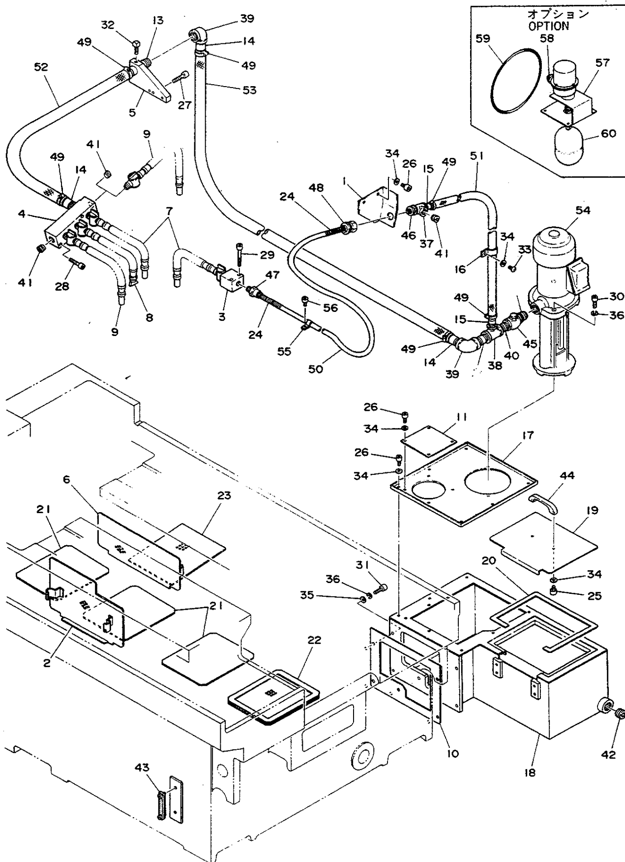
クーラント Fig.6I COOLANT
