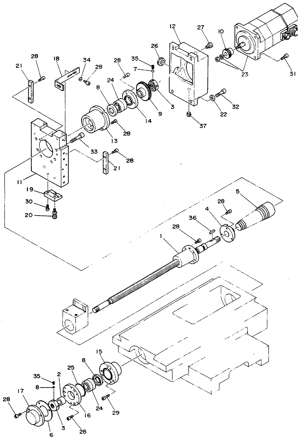
メインタレットスライド-5/7 Fig.5I MAIN TURRET SLIDE-5/7
