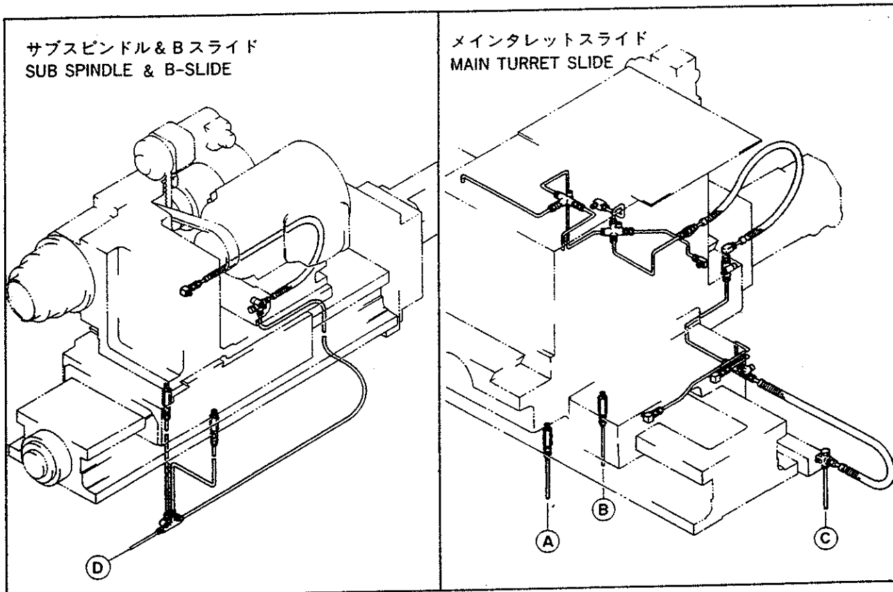
ルブリケイティングシステム Fig.63 LUBRICATING SYSTEM
