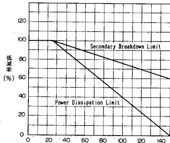
ケース温度 T_c ( ^\circ\text{C} ) ASO 低減特性 ASO Derating
