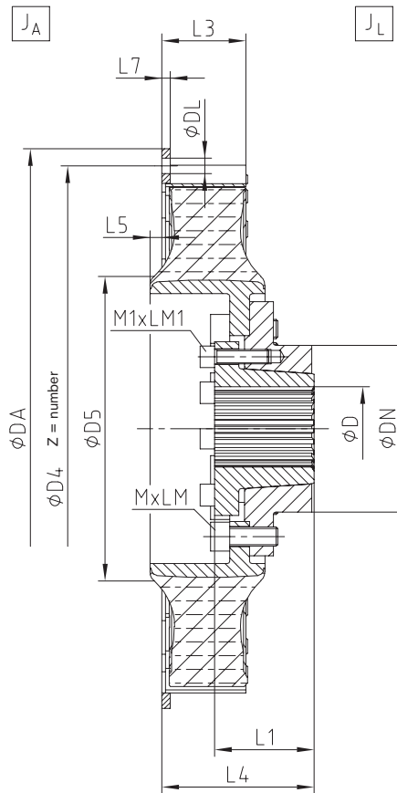
Type ALC
