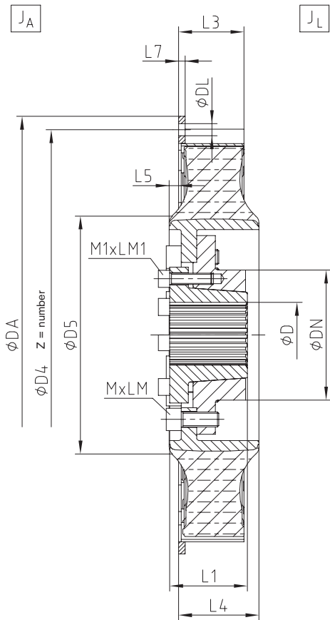
Type AKC
