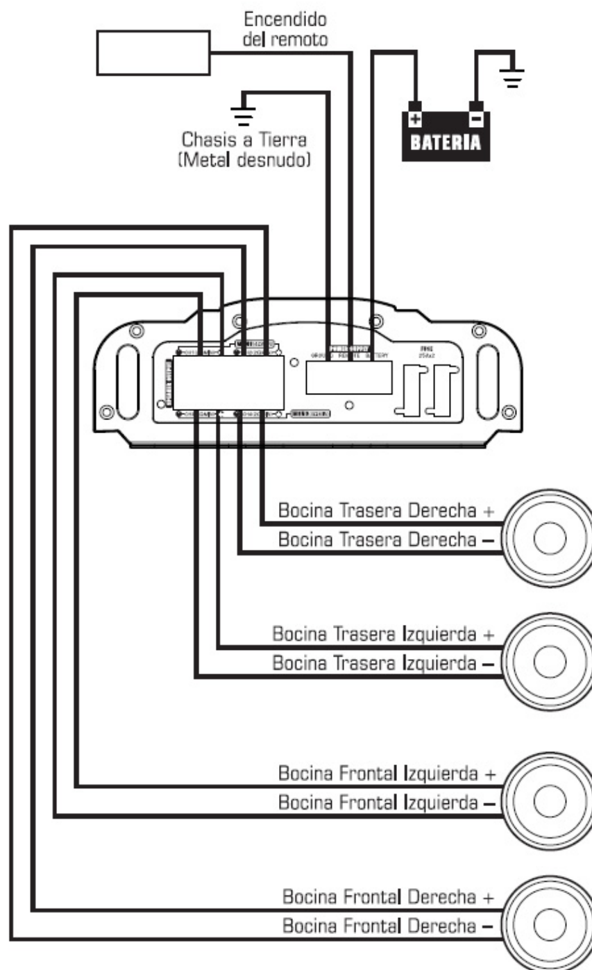
Figura 3 Conexiones para la potencia y las bocinas
