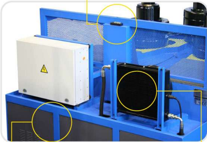
Painéis removíveis para fácil acesso ao grupo hidráulico Centralized hydraulic group for easy maintenance Paneles removibles para fácil acceso al grupo hidráulico
