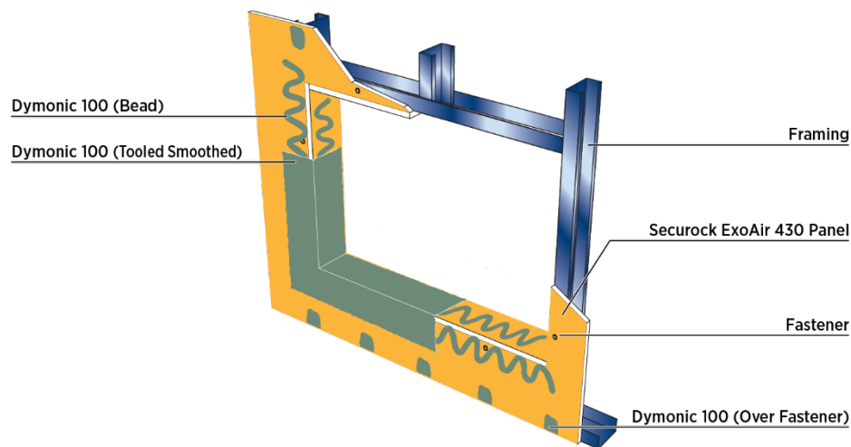
Fig. 7 : Rough Opening
