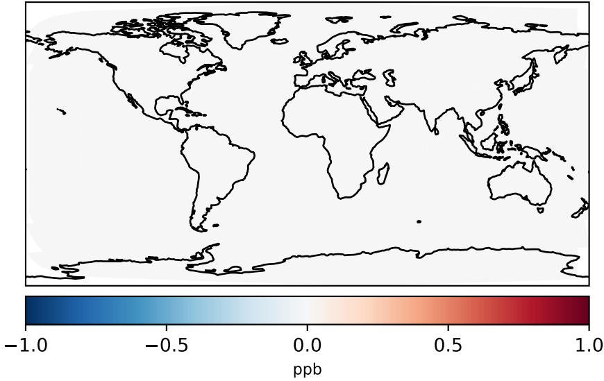
gchp-c24-1Mon-14.6.0-alpha.6_-_gchp-c24-1Mon-14.6.0-alpha.5 (Dev) c24
