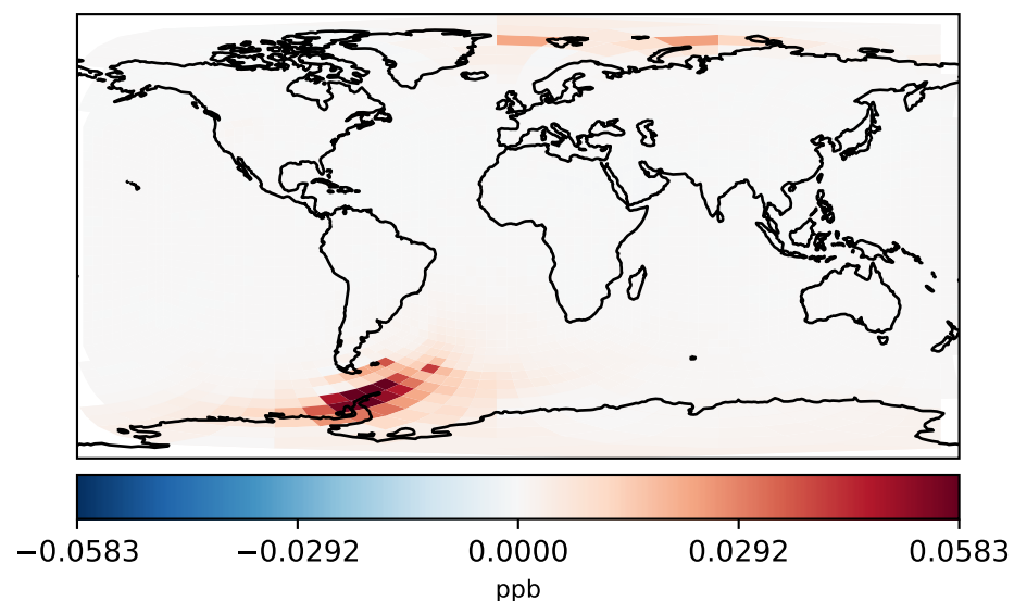
gchp-c24-1Mon-14.6.0-alpha.6_-_gchp-c24-1Mon-14.6.0-alpha.5 (Dev) c24
