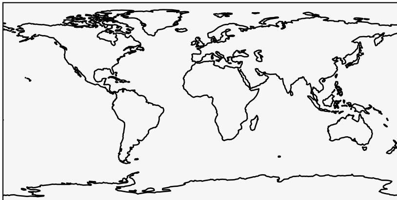
GCC_dev - GCC_ref (Ref) 4.0x5.0
