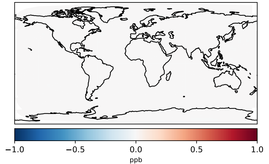
gchp-c24-1Mon-14.6.3_-_gchp-c24-1Mon-14.6.2 (Dev) c24
