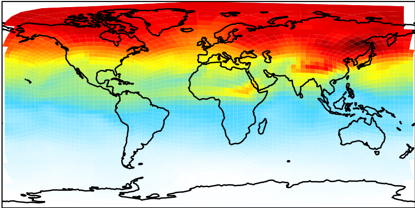
gchp-c24-1Mon-14.6.2 (Ref) c24
