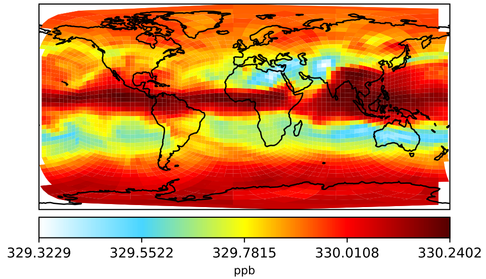
gchp-c24-1Mon-14.6.2 (Ref) c24
