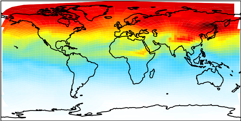
gchp-c24-1Mon-14.6.2 (Dev) c24
