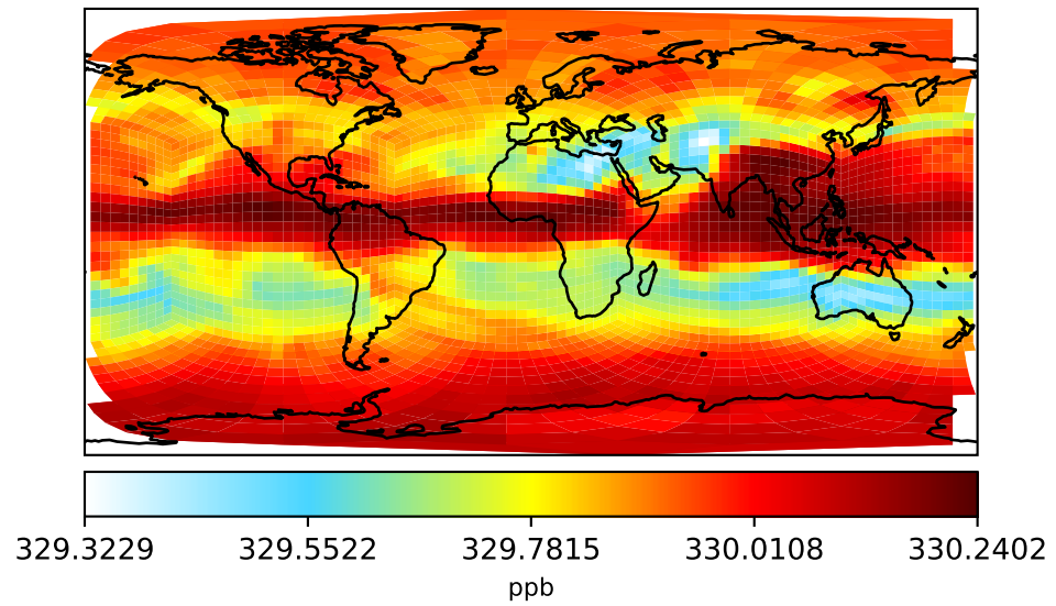
gchp-c24-1Mon-14.5.1 (Ref) c24
