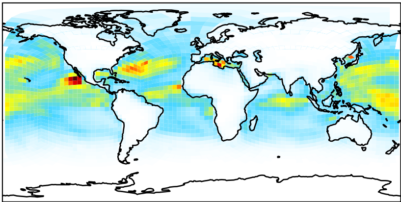
gchp-c24-1Mon-14.5.0-alpha.15 (Dev) c24
