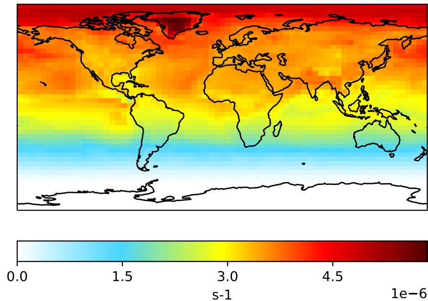
GCC_dev (Ref) 4.0x5.0
