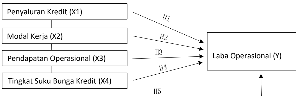
Gambar 1.1 Kerangka Konseptual
