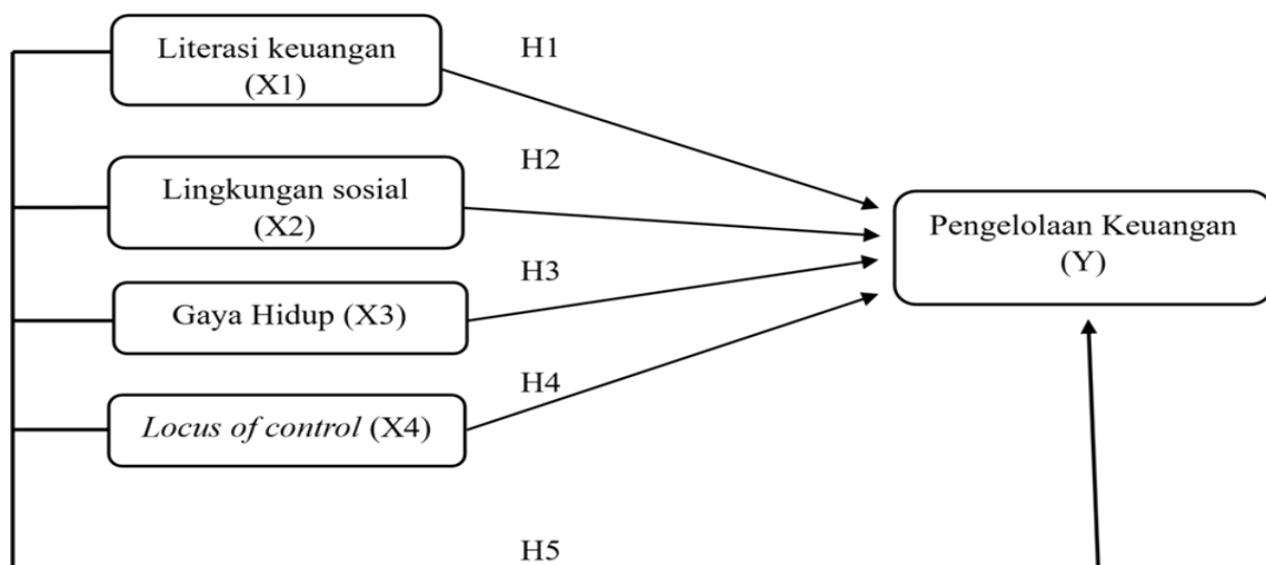
Gambar 1.1 Kerangka konseptual
