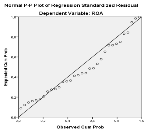
Gambar 3 Uji Normalitas P-P Plot Sumber : Hasil Pengolahan Data, 2020
