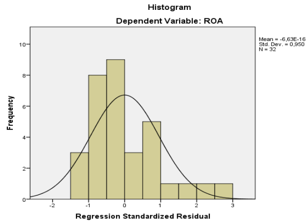
Gambar 2 Uji Grafik Histogram Sumber : Hasil Pengolahan Data, 2020
