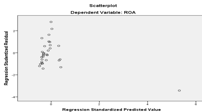
Gambar 4 Grafik Scatterplot Sumber : Hasil Pengolahan Data, 2020
