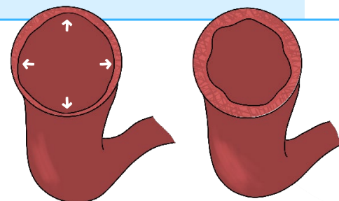
VASODILATION
