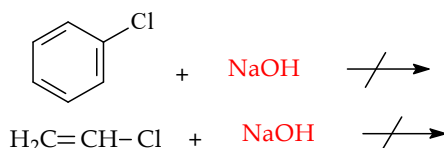
Gambar 6.34 Reaksi fenilklorida dan vinilklorida dengan NaOH
