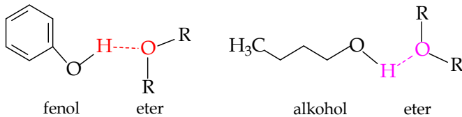
Gambar 8.13 Ikatan hidrogen antara eter dengan fenol dan alkohol
