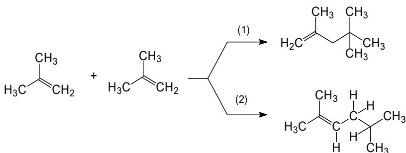
Gambar 4.28 Skema reaksi adisi antar senyawa alkena yang sejenis
