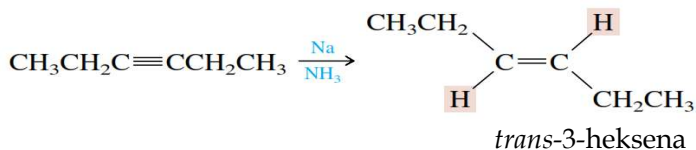
Gambar 5.17 Reaksi adisi hidrogenasi senyawa alkuna
