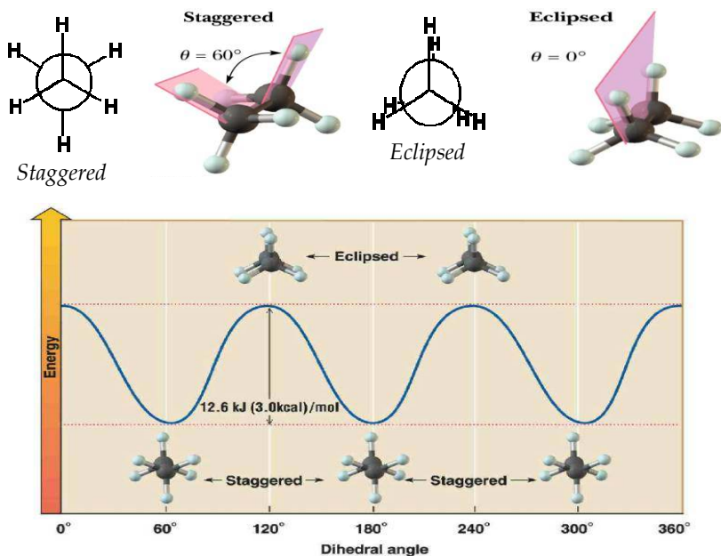
Gambar 2.25 Konformasi ekstrim dari etana, bersilang ( staggered ) dan berimpit ( eklips ) dan pola profil energinya
