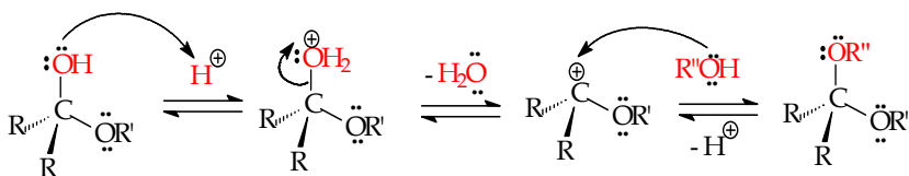
Gambar 10.36 Mekanisme pembentukan ketal 1
