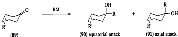
Gambar 3.46 Reaksi adisi terhadap senyawa sikloheksanon 13
