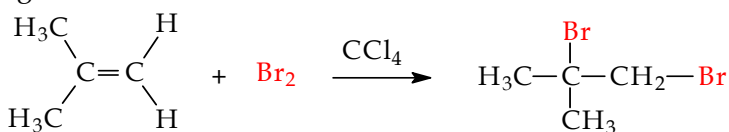
Gambar 4.23 Skema reaksi adisi halogenasi
