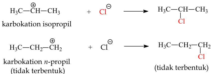
Gambar 4.37 Pembentukan karbokation isopropil
