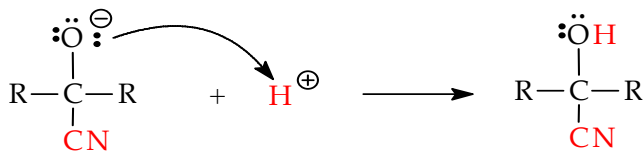
Gambar 10.21 Mekanisme adisi nukleofilik gugus karbonil dengan HCN (tahap 1)
