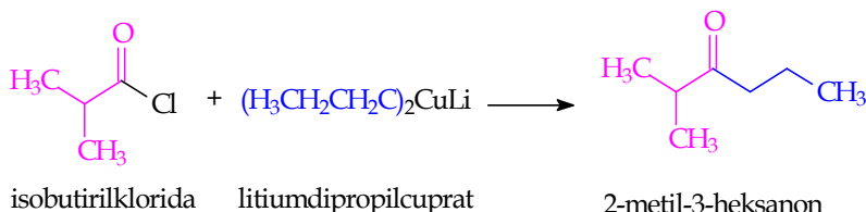
Gambar 10.68 Sintesis keton dari asilhalida dengan reagen R 2 CuLi
