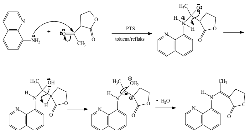
Gambar 10.54 Mekanisme reaksi sintesis senyawa 3-[1-(kuinolin-8-ilamino)-etiliden]-4,5-dihidro-furan-2-on
