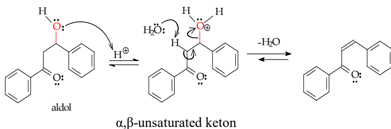
Gambar 10.71 Tahap dehidrasi dalam mekanisme enol
