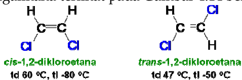
Gambar 4.14 Senyawa etena konfigurasi cis-trans
