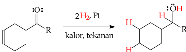
Gambar 10.46 Reduksi dengan hidrogenasi katalitik
