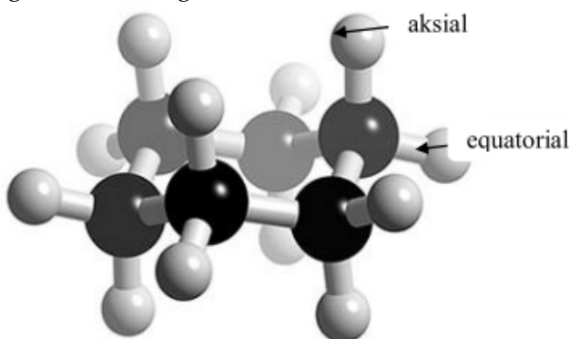
Gambar 3.18 Konformasi kursi sikloheksana menunjukkan posisi atom-atom hidrogen aksial dan ekuatorial
