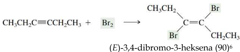
Gambar 5.34 Reaksi adisi halogenasi senyawa 3-heksuna 6
