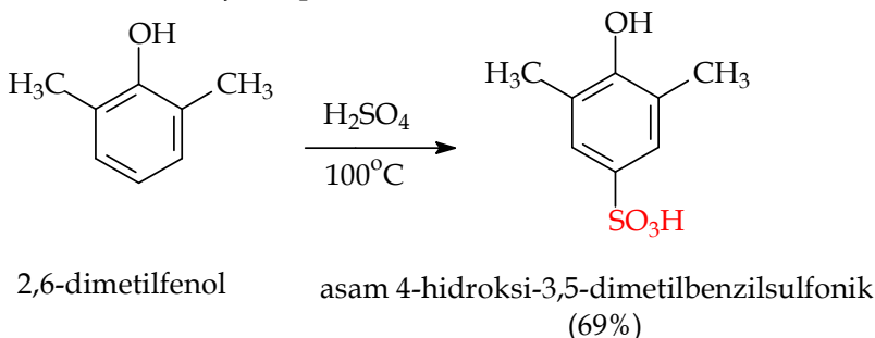
Gambar 7.35 Reaksi sulfonasi senyawa fenol
