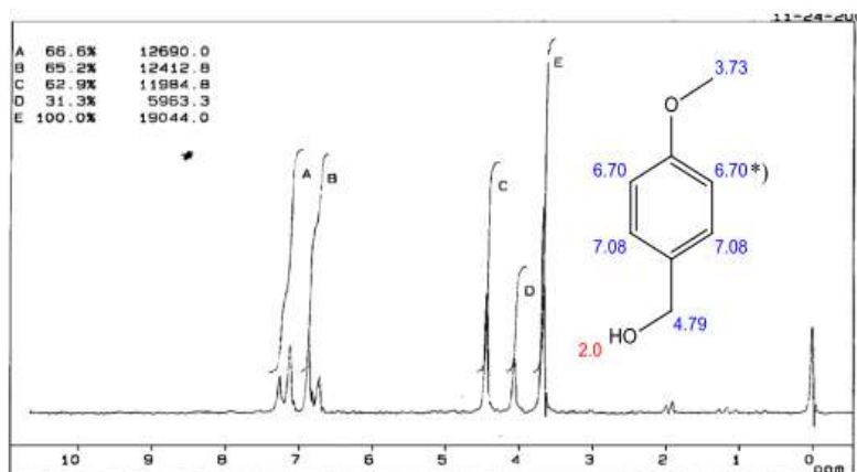
Gambar 9.53 Spektrum ^1\text{H} -NMR 4-metoksibenzil alkohol ( \text{CDCl}_3 , 60 MHz)
