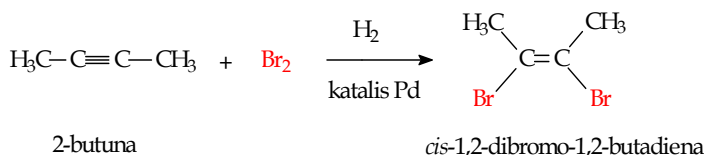
Gambar 5.15 Reaksi adisi senyawa alkuna
