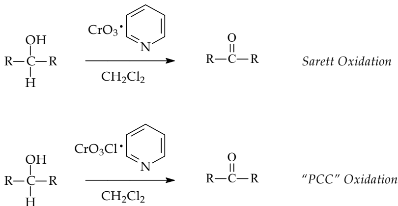
Gambar 6.24 Oksidasi alkohol dengan Pyridinium Chlorochromate
