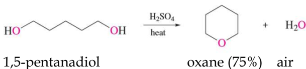
Gambar 8.27 Sintesis eter siklis oxane
