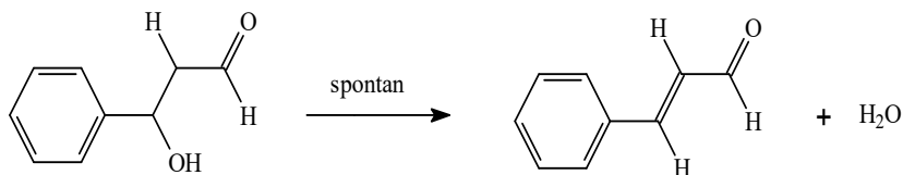
Gambar 9.70 Perubahan secara spontan dari 3-hidroksi-3-fenilpronaldehid ke sinmalaldehid 13
