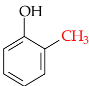
orto -metilfenol
