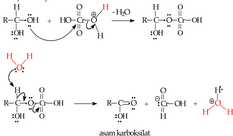
Gambar 6.23 Mekanisme oksidasi alkohol \text{H}_2\text{CrO}_4/\text{H}_2\text{SO}_4 menjadi asam karboksilat
