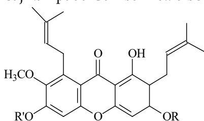
Gambar 10.90 Struktur molekul senyawa turunan mangostin
