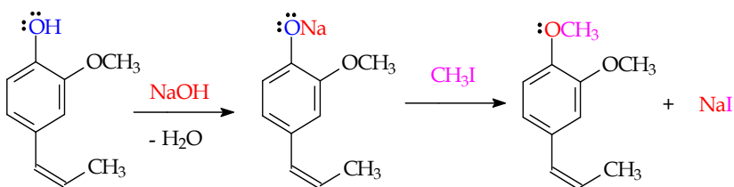
Gambar 7.28 Skema reaksi pembentukan ion eugenoksida
