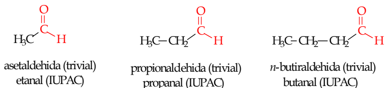
Gambar 9.3 Tata nama senyawa aldehid sederhana
