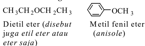
Gambar 8.7 Penamaan eter sederhana
