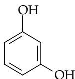
resorcinol 1,3-benzenadiol
