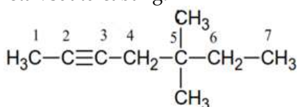
Gambar 5.6 Penentuan rantai utama 5,5-dimetil-2-heptuna
