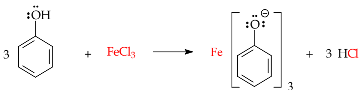
Gambar 7.29 Reaksi fenol dengan \text{FeCl}_3
