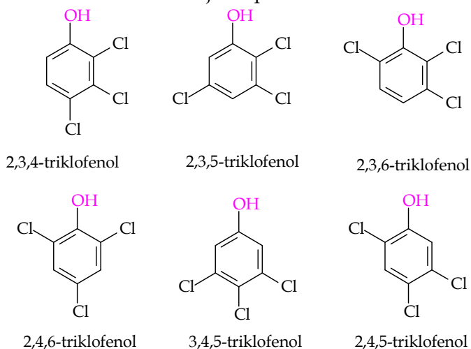
Gambar 7.44 Isomer fenol yang memiliki 3 substituen gugus lain
