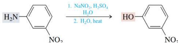
Gambar 7.38 Reaksi sintesis m -nitrofenol dari m -nitroanilin
