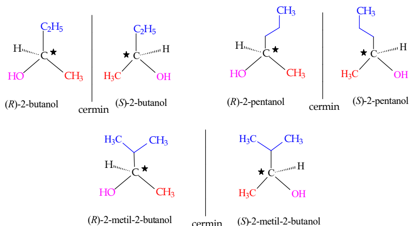
Gambar 6.60 Isomeri konfigurasi senyawa alkohol
