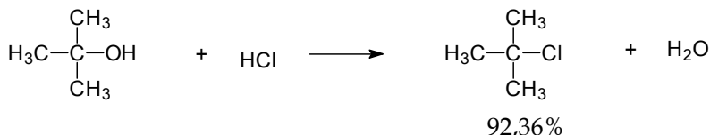
Gambar 6.27 Reaksi t -butialkohol dengan asam klorida 6
