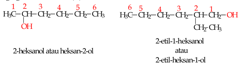
Gambar 6.2 Tata nama senyawa alkohol
