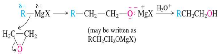
Gambar 8.20 Reaksi senyawa epoksida dengan reagen Grignard 4
