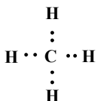
metana
