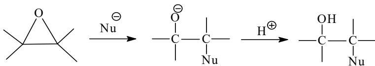
Gambar 8.17 Mekanisme reaksi epoksida dengan asam halida
