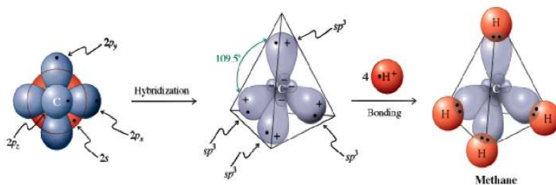
Gambar 1.9 Hibridisasi sp^3 pada metana
