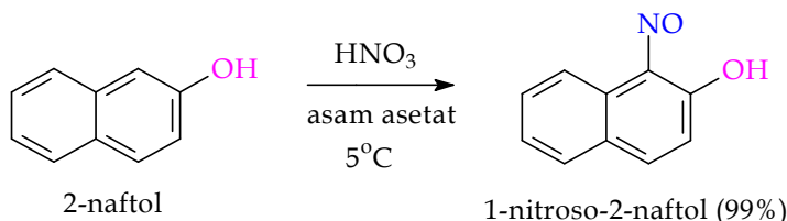
Gambar 7.33 Reaksi nitrosasi senyawa fenol dengan asam nitrat
