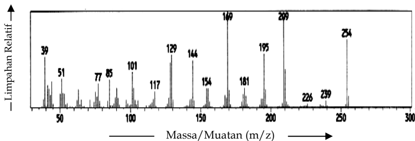
Gambar 10.57 Spektrum massa senyawa 3-[1-(kuinolin-8-ilamino)-etiliden]-4,5-dihidrofuran-2-on 8
