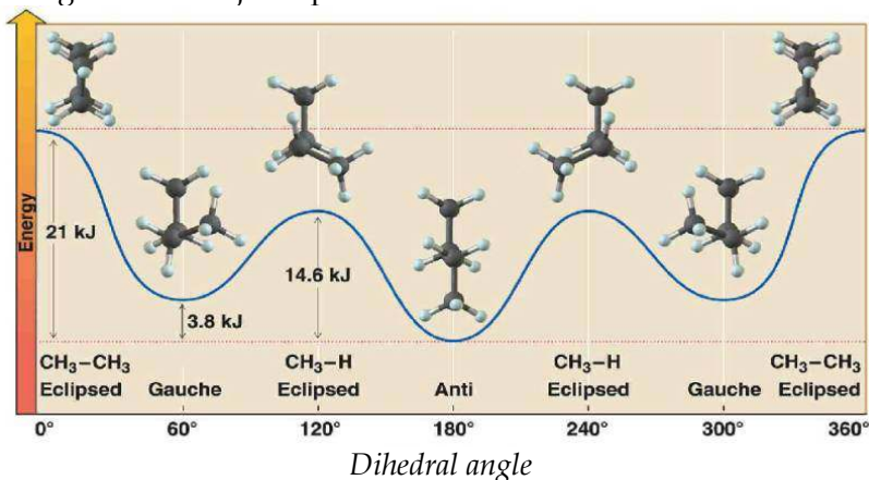
Gambar 2.27 Hubungan energi dengan berbagai konformasi n -butana
