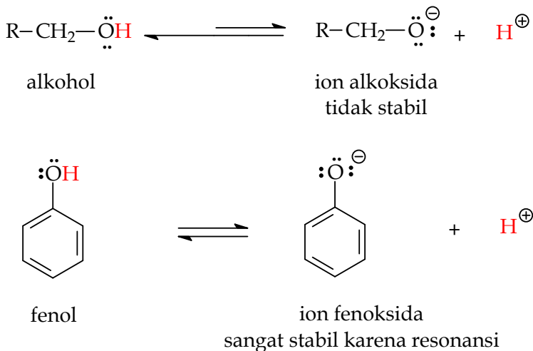
Gambar 7.15 Struktur ionisasi senyawa fenol
