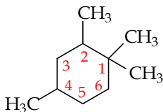
1,1,2,4-tetrametilsikloheksana
