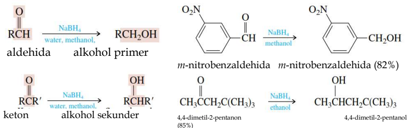
Gambar 6.49 Reaksi reduksi aldehyd atau keton dengan reagen \text{NaBH}_4
