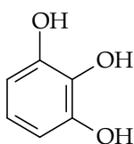
pyragallol 1,2,3-benzenatriol
