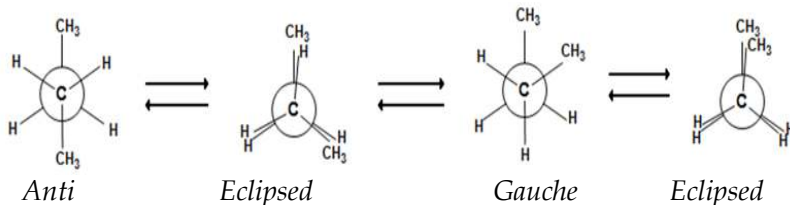
Gambar 2.26 Konformasi senyawa n -butana
