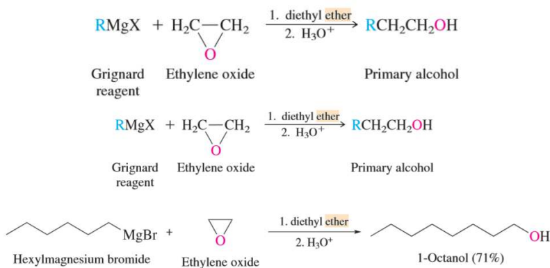
Gambar 8.19 Reaksi senyawa epoksida dengan reagen Grignard 4
