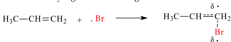
Gambar 4.44 Keadaan transisi pada reaksi adisi radikal bebas
