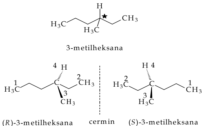
Gambar 2.12 Stereoisomer senyawa 3-metilheksana
