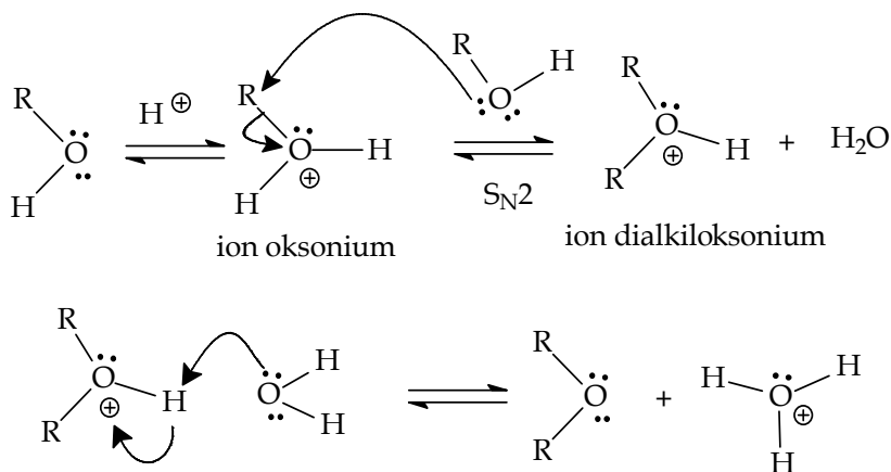
Gambar 8.22 Mekanisme reaksi umum sintesis senyawa eter
