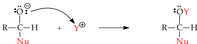
Gambar 9.28 Mekanisme reaksi adisi nukleofilik pada karbonil 4
