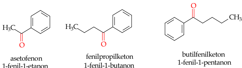
Gambar 10.3 Senyawa alkil aril keton
