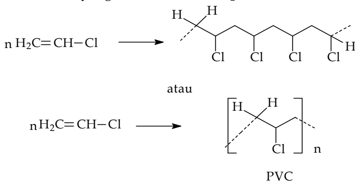
Gambar 4.9 Reaksi polimerisasi terhadap senyawa alkena
