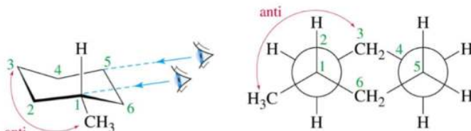
Gambar 3.17. Proyeksi Newman senyawa sikloheksana 3
