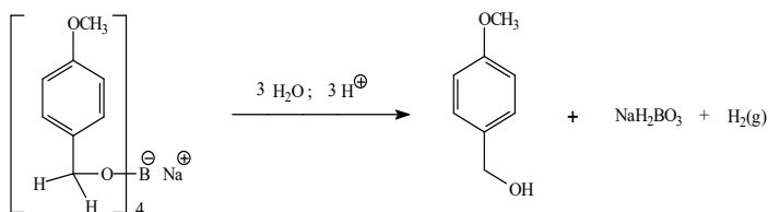
Gambar 6.53 Mekanisme reaksi tahap 2 reduksi 4-metoksibenzaldehid
