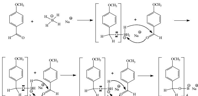
Gambar 6.52 Mekanisme reaksi tahap 1 reduksi 4-metoksibenzaldehid
