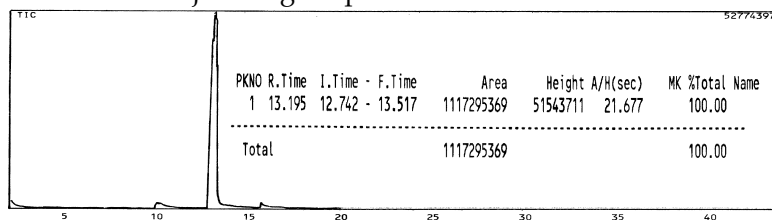
Gambar 9.72 Kromatogram senyawa sinmalaldehid
