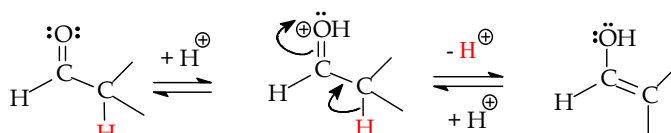
Gambar 9.14 Perubahan bolak-balik asetal-enol katalis asam
