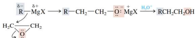
Gambar 6.57 Mekanisme reaksi etilen oksida dengan reagen Grignard
