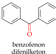
Gambar 10.4 Senyawa keton aromatik
