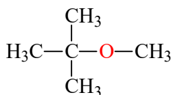
Gambar 8.28 Struktur senyawa MTBE
