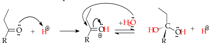
Gambar 10.42 Mekanisme reaksi pada kondisi asam
