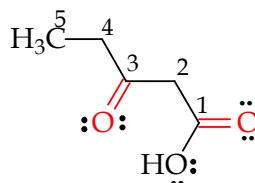
asam 3-oksopentanoat
