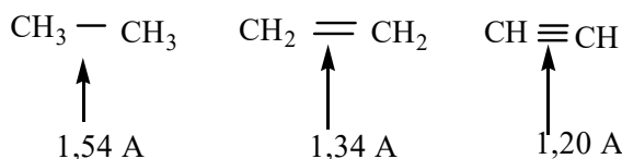
Gambar 5.2 Perbandingan panjang ikatan karbon-karbon 5
