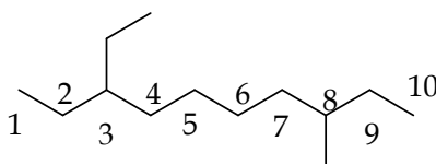
3-etil-8-metildekana
