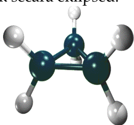
Gambar 3.9 Siklopropana, dengan model bola-tongkat
