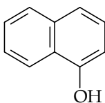
naphthalen-1-ol
