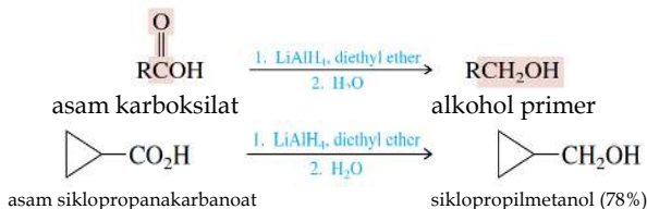
Gambar 6.54 Reaksi reduksi asam karboksilat menggunakan \text{NaBH}_4
