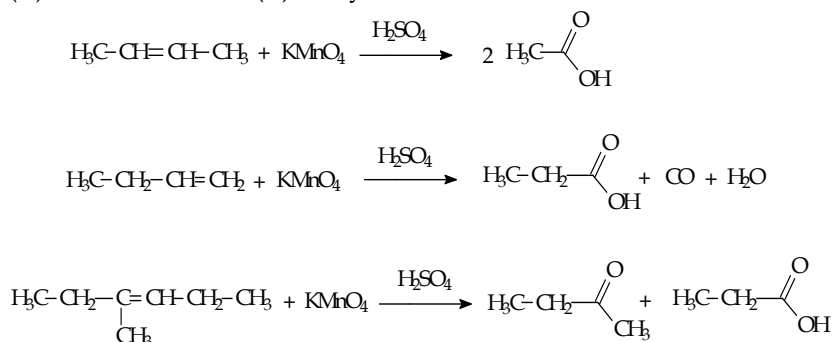
Gambar 4.11 Reaksi oksidasi senyawa alkena dengan \text{KMnO}_4
