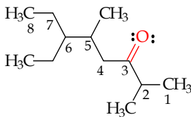
6-etil-2,5-dimetil-3-butanon
