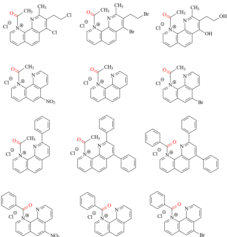
Gambar 10.86 Struktur karbonil turunan 1,10-fenantrolin
