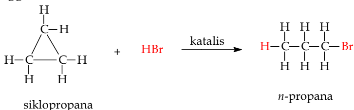
Gambar 3.39 Reaksi brominasi terhadap siklopropana
