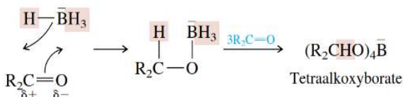
Gambar 6.50 Mekanisme awal reaksi reduksi dengan \text{NaBH}_4
