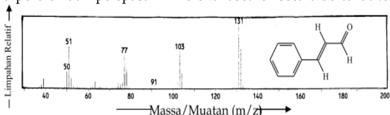
Gambar 9.74 Spektrum massa sinmalaldehid (Puncak 4) (EI)
