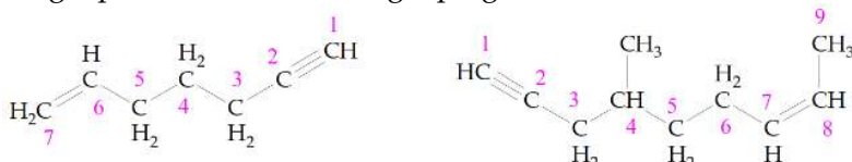
1-hepten-6-una/6-hepten-1-una 4-metil-7-nonen-1-una
