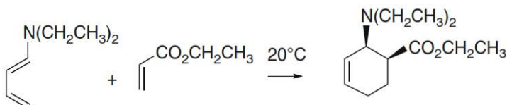
Gambar 3.50 Pembentukan cincin sikloheksena 16
