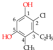
3-etil-2-kloro-4-metil-1,5-dihidroksi-benzena
