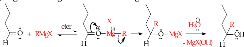
Gambar 9.42 Adisi senyawa aldehyd dengan pereaksi Grignard
