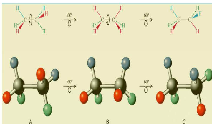
Gambar 2.24 Konformasi senyawa etana
