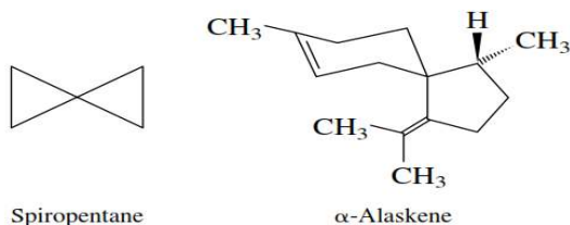
Gambar 3.32 Struktur senyawa spirosiklik: spiropentana dan α-alasken 3
