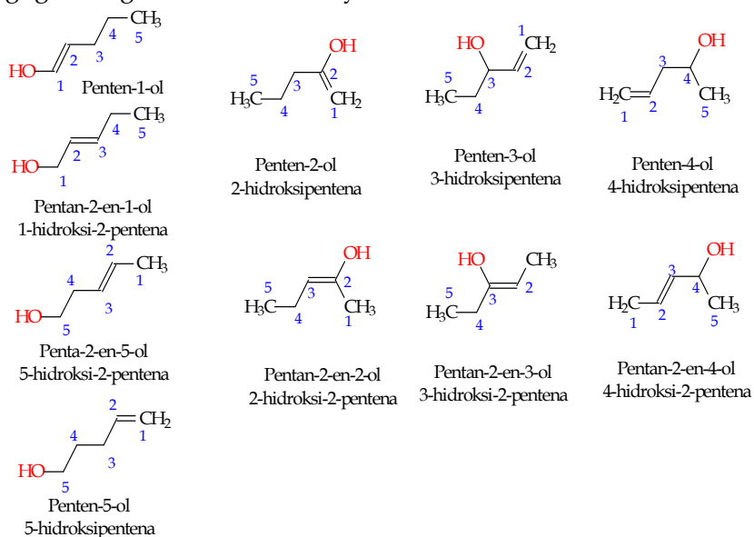
Gambar 10.79 Semua isomer gugus fungsi dari C_5H_{10}O
