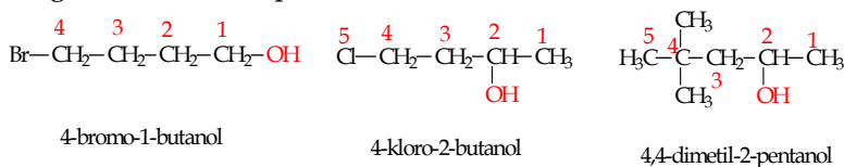
Gambar 6.3 Penomoran atom karbon senyawa alkohol
