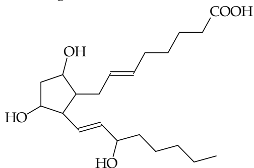
Gambar 3.51 Senyawa turunan siklopentana PGF 2α
