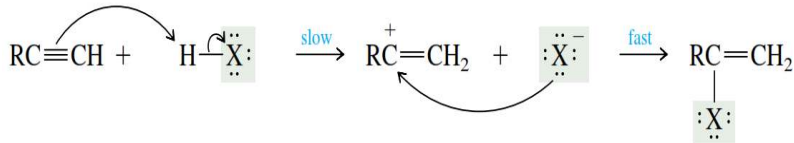
Gambar 5.27 Mekanisme reaksi adisi hidrohalogenasi senyawa alkuna 6
