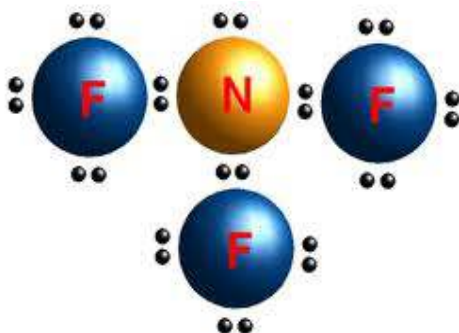
Gambar 1.3 Struktur Lewis
