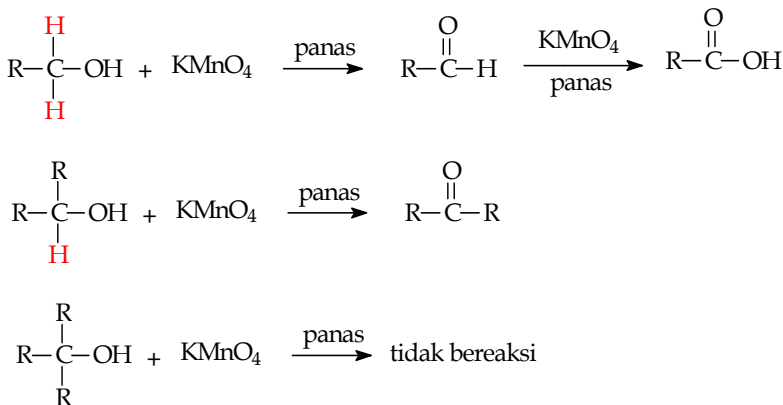
Gambar 6.20 Oksidasi senyawa alkohol dengan \text{KMnO}_4
