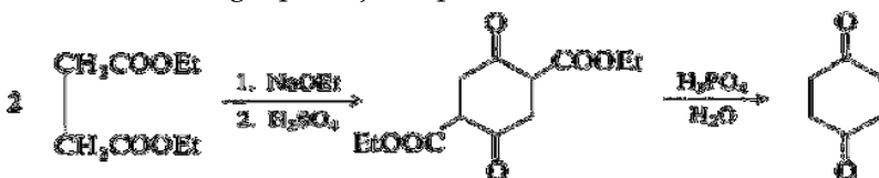
Gambar 3.42 Sintesis senyawa 1,4-sikloheksanadion 15
