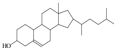
kolesterol (suatu steroid)
