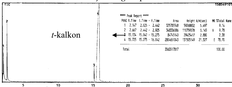
Gambar 10.76 Kromatogram senyawa t -kalkon
