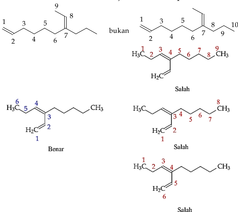
Gambar 4.1 Cara penomoran dan penentuan rantai induk
