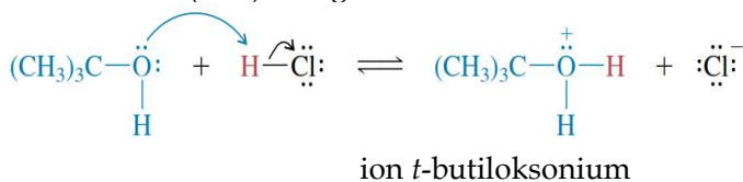
Gambar 6.28 Protonasi senyawa t -butilalkohol 2
