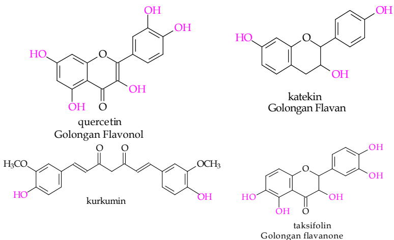
Gambar 7.8 Senyawa quersitin, katekin, kurkumin, dan taksifolin
