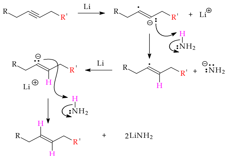
Gambar 5.40 Mekanisme reaksi adisi senyawa alkuna dengan Li dan NH 3
