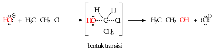
Gambar 6.33 Mekanisme reaksi alkil halida menjadi alkohol
