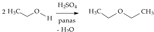
Gambar 8.21 Sintesis senyawa dietil eter
