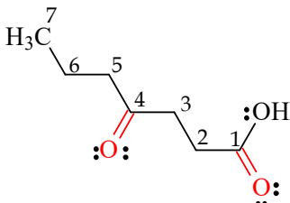
asam 4-oksoheptanoat
