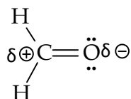
Gambar 9.36 Muatan parsial senyawa formaldehid
