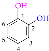
Gambar 7.2 Struktur senyawa 1,2-benzenadiol (pyrokatekol)
