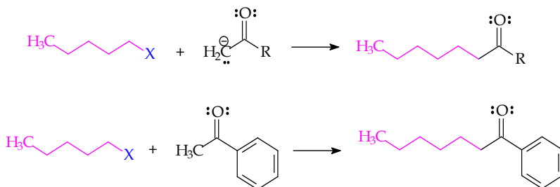
Gambar 10.65 Reaksi sintesis keton dengan R lebih panjang
