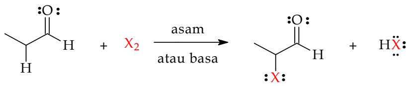
Gambar 9.58 Skema umum reaksi halogenasi senyawa aldehid
