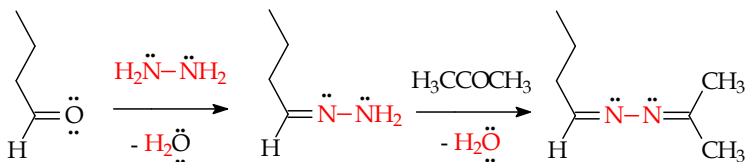
Gambar 9.47 Reaksi kondensasi aldehid dengan hidrazin 9
