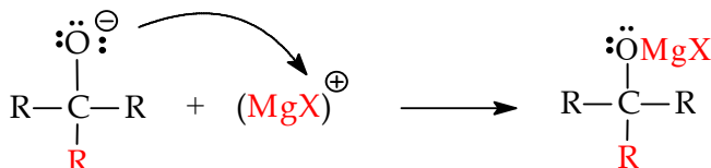
Gambar 10.24 Mekanisme adisi gugus karbonilpereaksi Girgnard (tahap 2)
