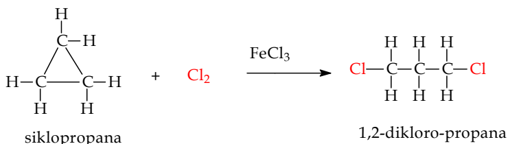
Gambar 3.37 Reaksi klorinasi senyawa siklopropana
