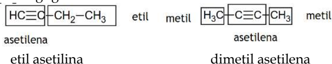
Gambar 5.11 Nama trivial alkuna sederhana
