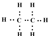
etana
