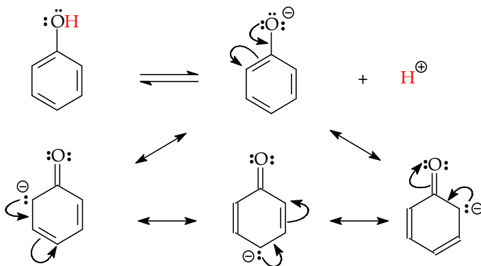
Gambar 7.16 Struktur resonansi ion fenoksida
