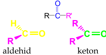
Gambar 10.10 Perbedaan struktur aldehid dan keton
