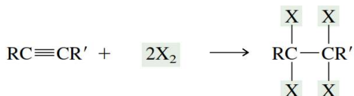
Gambar 5.33 Kerangka umum reaksi adisi halogenasi 6
