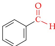
Gambar 9.1 Kerangka struktur senyawa aldehyd
