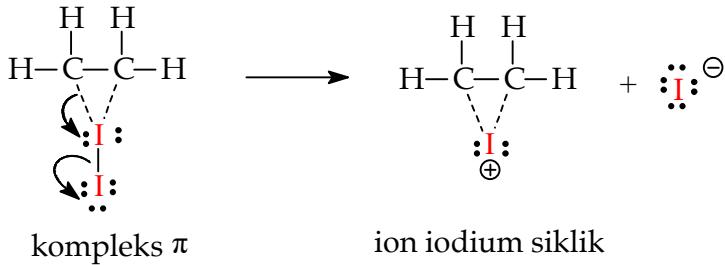
Gambar 4.33 Langkah 2 mekanisme reaksi iodinasi
