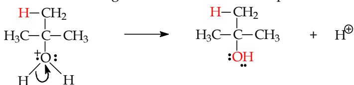
Gambar 4.40 Langkah 3 mekanisme hidrasi pada alkena
