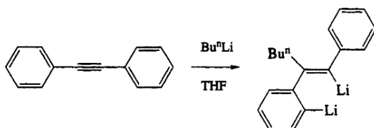
Gambar 5.35 Reaksi adisi senyawa alkuna khususnya 1,2-difeniletuna 9
