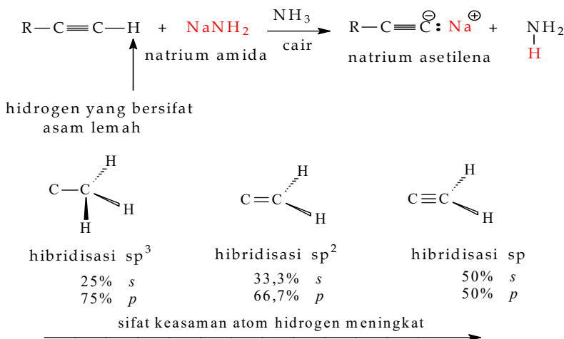
Gambar 5.13 Reaksi senyawa alkuna dengan natrium amida
