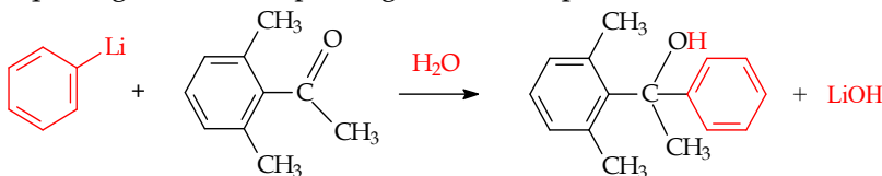
Gambar 6.41 Reaksi keton dengan organologam Pereaksi Grignard dengan etilen oksida.
