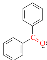
difenilketon
