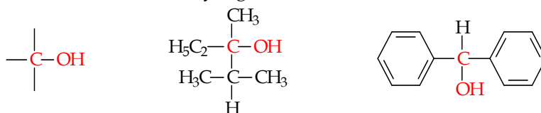
Gambar 6.6 Penamaan turunan metanol atau karbinol
