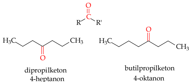
Gambar 10.2 Senyawa keton alifatik
