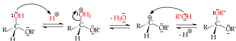
hemiasetal
