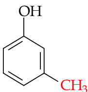
meta -metilfenol
