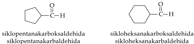
Gambar 9.6 Tata nama aldehid dengan akhiran karboksaldehid atau karbaldehid
