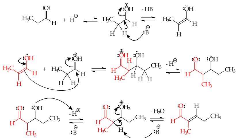
Gambar 9.67 Reaksi kondensasi aldol terkatalis asam
