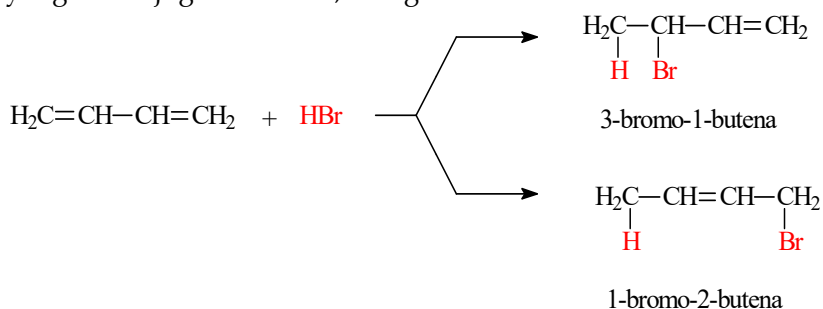
Gambar 4.29 Skema reaksi adisi pada diena terkonjugasi
