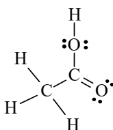
Gambar 1.6 Struktur Lewis asam asetat
