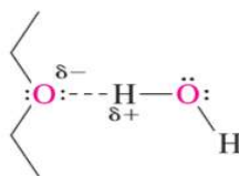
Gambar 8.12 Ikatan hidrogen senyawa eter
