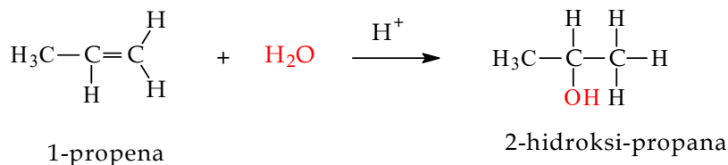
Gambar 4.21 Reaksi hidrasi
