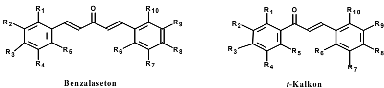
Gambar 10.84 Struktur turunan benzalaseton dan t -kalkon
