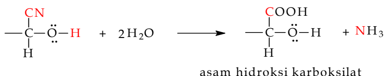
Gambar 9.21 Sintesis asam hidroksi karboksilat dari bahan baku aldehid
