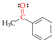
asetofenon
