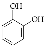
pyrochatecol 1,2-benzenadiol
