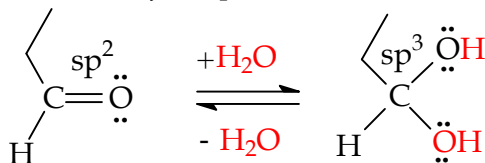
Gambar 9.34 Serangan gugus karbon karbonil terhadap nukleofil
