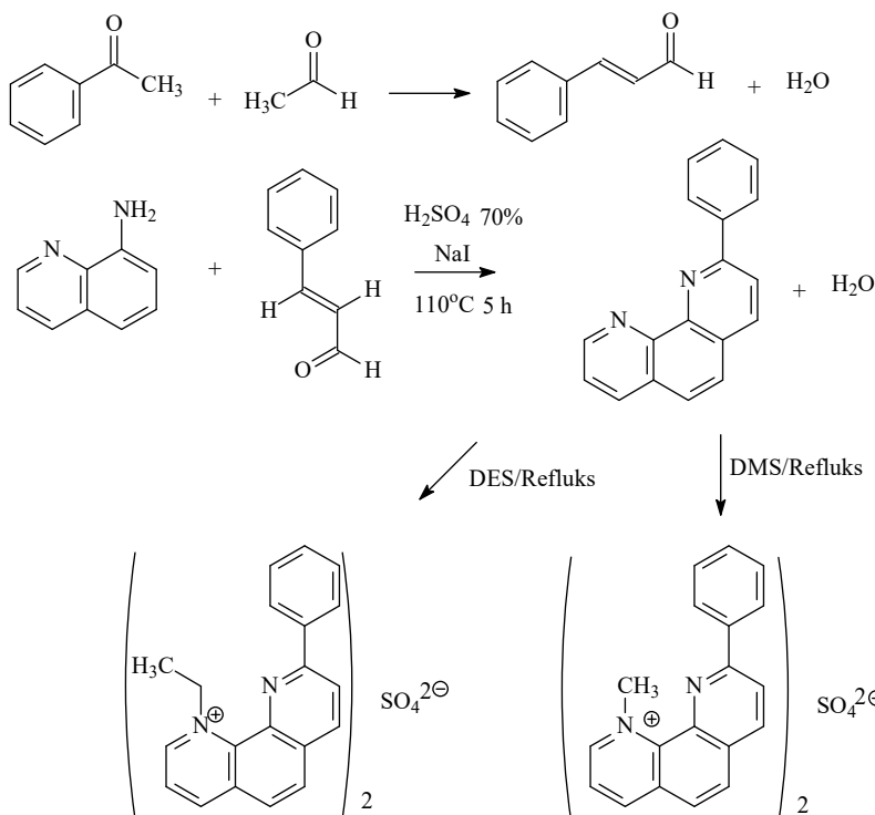
Gambar 10.96 Reaksi sintesis (1)-N-metil-9-fenil-1,10-fenantrolinium sulfat dan (1)-N-etil-9-fenil-1,10-fenantrolinium sulfat dari bahan dasar karbonil
