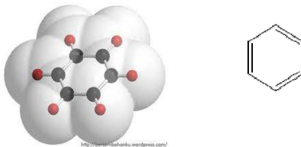
Gambar 1.23 Struktur Kekule senyawa benzena
