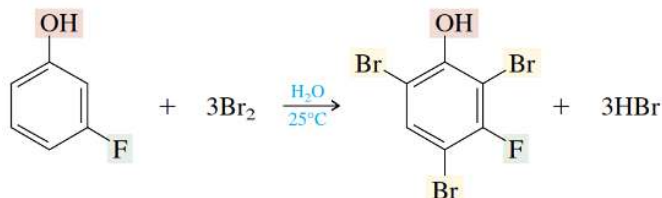
Gambar 7.26 Reaksi brominasi senyawa m -florofenol 1
