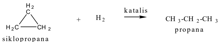
Gambar 3.38 Reaksi hidrogenasi terhadap siklopropana
