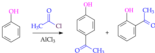
Gambar 7.30 Reaksi asilasi senyawa fenol dengan asil klorida
