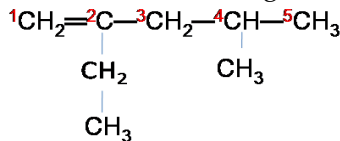
2-etil-4-metil-1-pentena
