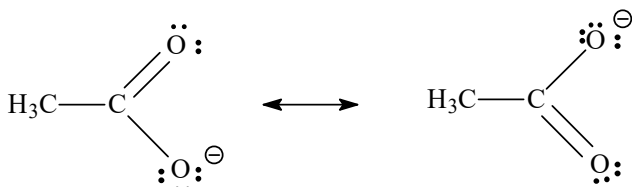
Gambar 1.37 Struktur resonansi dari anion asetat
