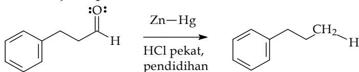
Gambar 9.55 Reduksi gugus aldehid menjadi gugus metilen
