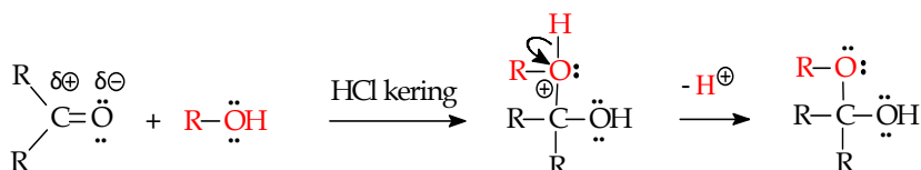
Gambar 10.34 Adisi gugus karbonil dengan pereaksi alkohol
