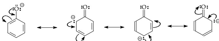
Gambar 7.19 Struktur resonansi ion fenoksida 1
