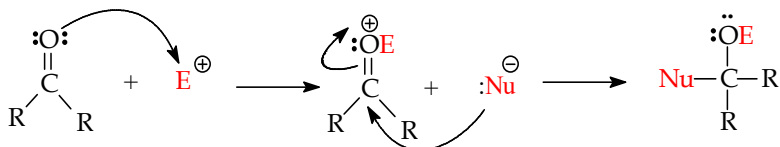
Gambar 9.33 Serangan gugus karbon karbonil terhadap nukleofil
