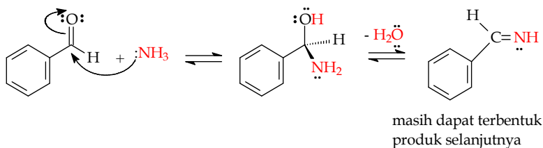
Gambar 9.44 Kondensasi aldehid dengan amoniak/turunannya
