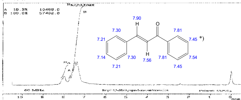
Gambar 10.75 Spektrum ^1\text{H-NMR} t -kalkon ( \text{CDCl}_3 , 60 MHz)
