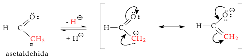
Gambar 9.11 Bentuk resonansi senyawa asetaldehid
