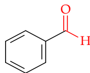
Gambar 9.2 Klasifikasi senyawa aldehyd
