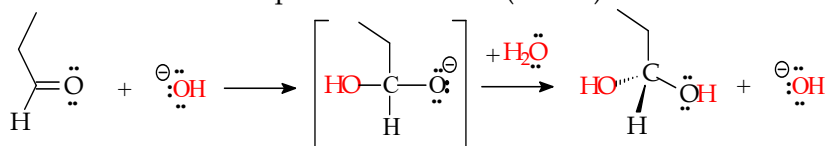
Gambar 9.39 Mekanisme reaksi kondisi basa adisi nukleofilik
