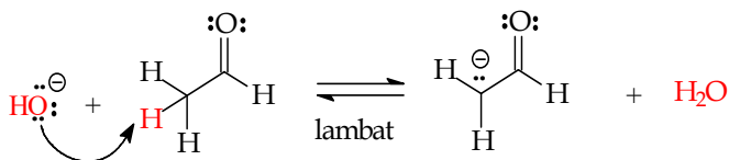
Gambar 9.62 Tahap satu mekanisme reaksi kondensasi aldol terkatalis basa
