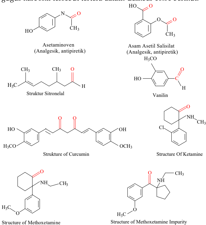
Gambar 10.81 Struktur senyawa obat bergugus karbonil
