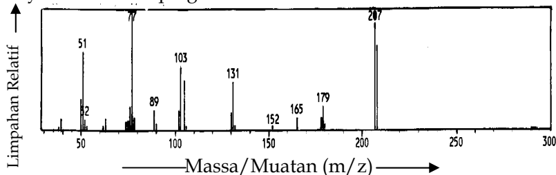
Gambar 10.77 Spektrum massa senyawa t -kalkon (EI)
