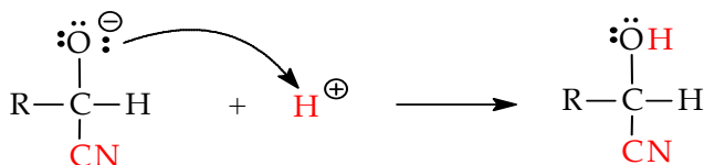
Gambar 9.22 Mekanisme adisi HCN pada aldehid 4,8
