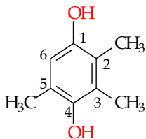
2,3,5-trimetil-1,4-dihidroksi-benzena
