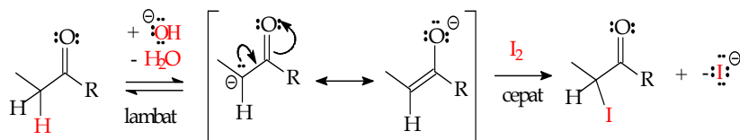
Gambar 10.50 Mekanisme reaksi halogenasi keton terkatalis basa
