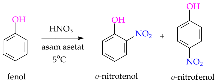
Gambar 7.25 Reaksi nitrasi senyawa fenol
