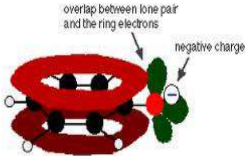
Gambar 7.17 Overlap pasangan elektron bebas dari oksigen dengan elektron dari rantai benzena
