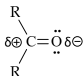
Gambar 10.16 Polarisasi muatan gugus karbonil
