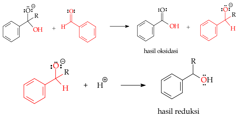
Gambar 10.39 Mekanisme reaksi Cannizzaro pada senyawa keton
