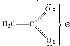
Gambar 1.36 Struktur hibrida resonansi (kanonik) dari anion asetat
