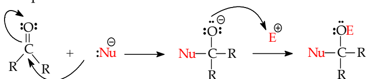
Gambar 10.18 Mekanisme adisi nukleofilik gugus keton 6
