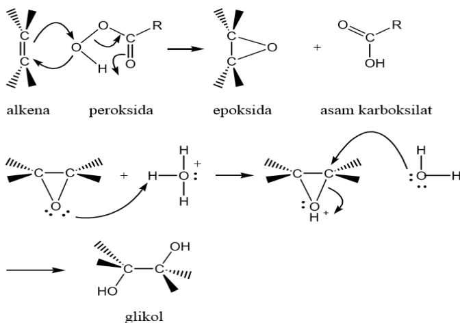
Gambar 8.15 Mekanisme reaksi epoksidasi senyawa alkena
