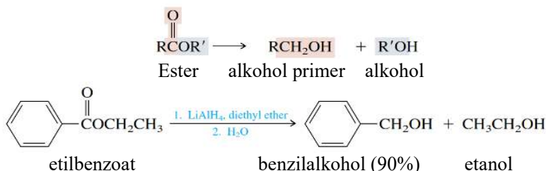
Gambar 6.55 Reduksi senyawa ester menggunakan reagen \text{LiAlH}_4
