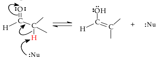
Gambar 9.15 Transfer proton senyawa asetaldehid 4
