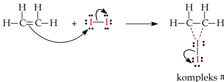
Gambar 4.32 Langkah 1 mekanisme reaksi iodinasi
