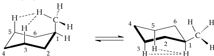
Gambar 3.19 Gugus metil dalam derajat ekuatorial (95%) dan aksial (5%) 3
