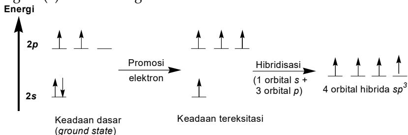
Gambar 1.7 Diagram energi hibridisasi pembentukan ikatan tunggal
