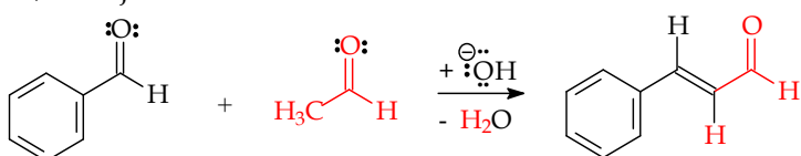
Gambar 9.66 Reaksi kondensasi senyawa aldol aromatis
