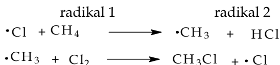
Gambar 2.32 Tahap propagasi pada reaksi klorinasi metana
