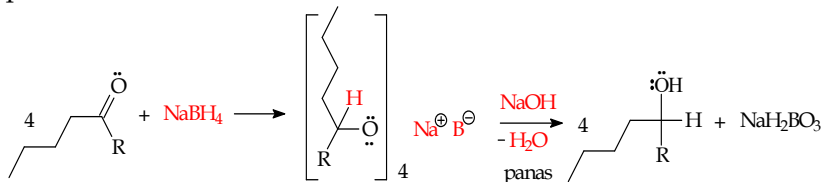
Gambar 10.45 Reduksi keton dengan \text{NaBH}_4
