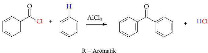
Gambar 10.62 Sintesis keton melalui asilasi Friedel-Crafts
