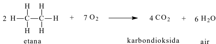
Gambar 2.34 Reaksi pembakaran etana
