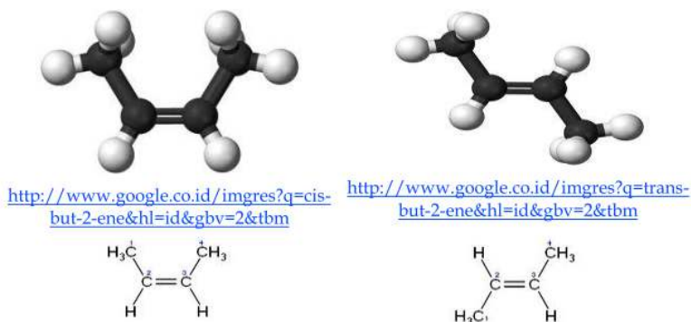
Gambar 4.13 Senyawa alkene konfigurasi cis-trans buten-2-ena model bola dan tongkat
