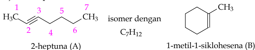
Gambar 5.46 Isomer gugus fungsi senyawa alkuna
