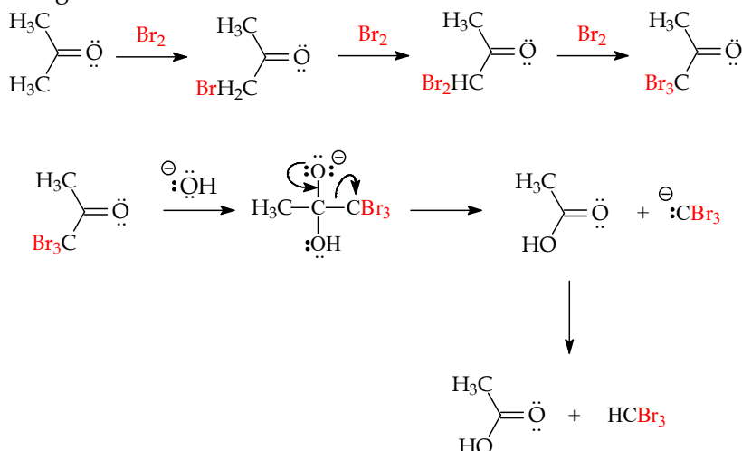
Gambar 10.52 Oksidasi keton kondisi halogen berlebihan
