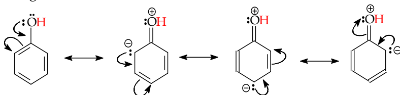
Gambar 7.20 Struktur resonansi senyawa fenol
