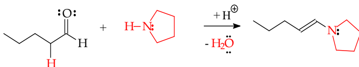
Gambar 9.46 Sintesis enamina bahan baku aldehid sekunder
