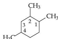
1,2,4-trimetilsikloheksana
