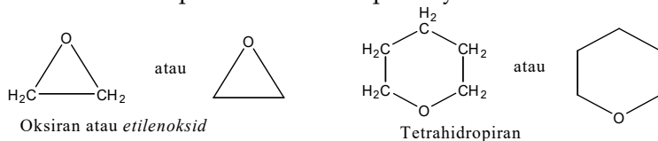
oxasiklopropana
